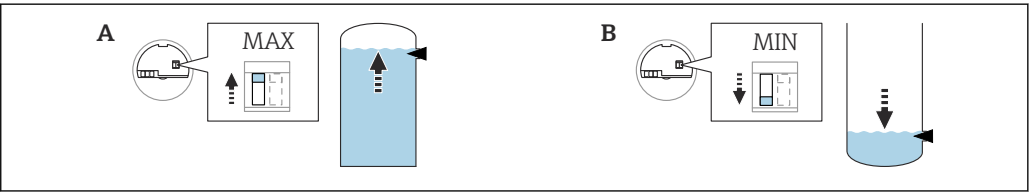
图 56 电子插件上的高限（MAX）/低限（MIN）检测开关位置
