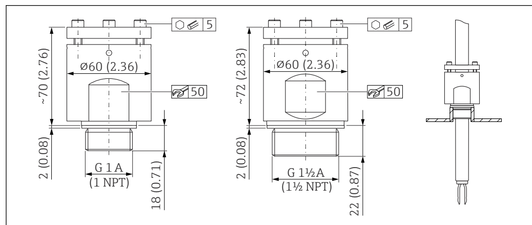
图 67 高压滑动套管。测量单位 mm (in)
