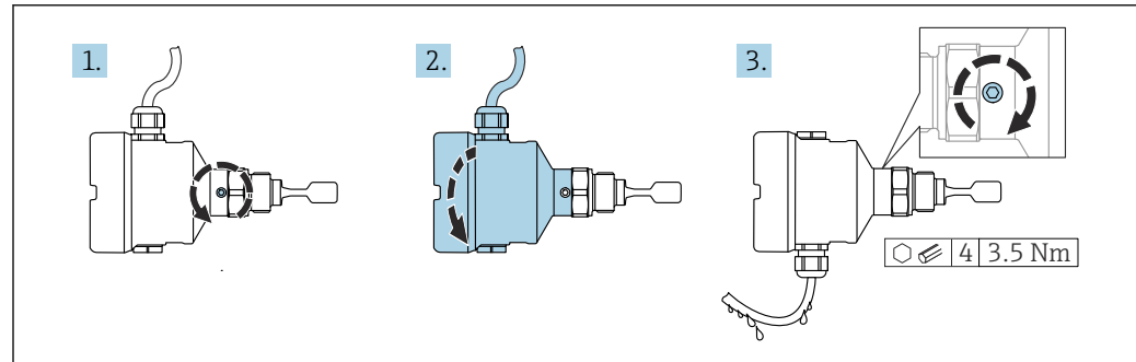
图 27 外壳带固定螺丝；在电缆上建立排水回路
