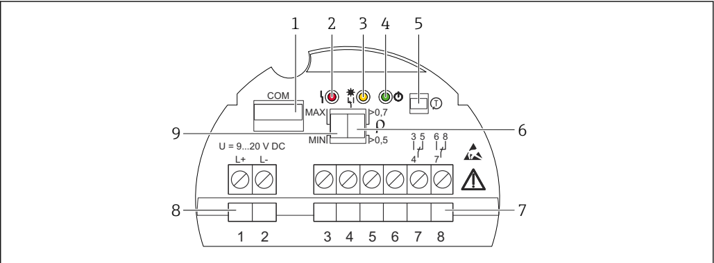
图 55 实例：电子插件 FEL64DC
