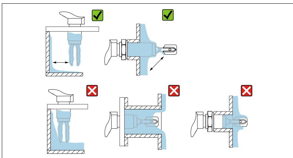
图 22 安装实例：测量高粘度过程介质
