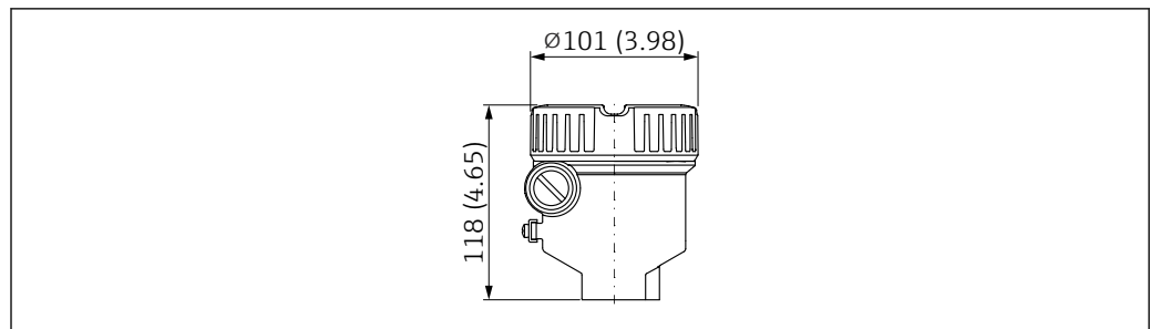
图 36 单腔体 316L 外壳的外形尺寸示意图；Ex d/XP、粉尘防爆场合；外壳盖不带观察窗。测量单位 mm (in)
