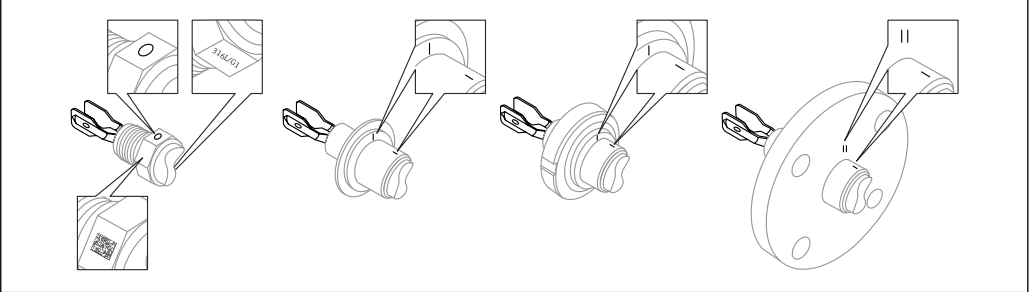
图 24 参照标记水平安装在罐体中时的音叉位置
