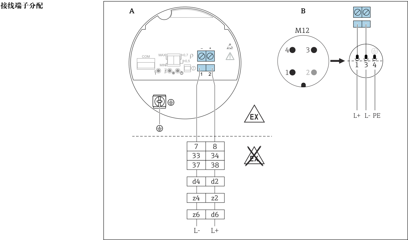
图 11 电子插件 FEL67：PFM 输出
