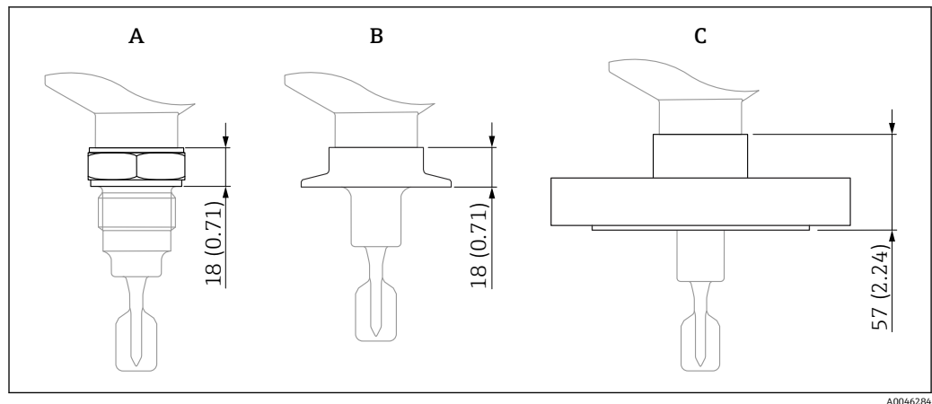
图 43 过程连接的最大高度规格。测量单位 mm (in)
