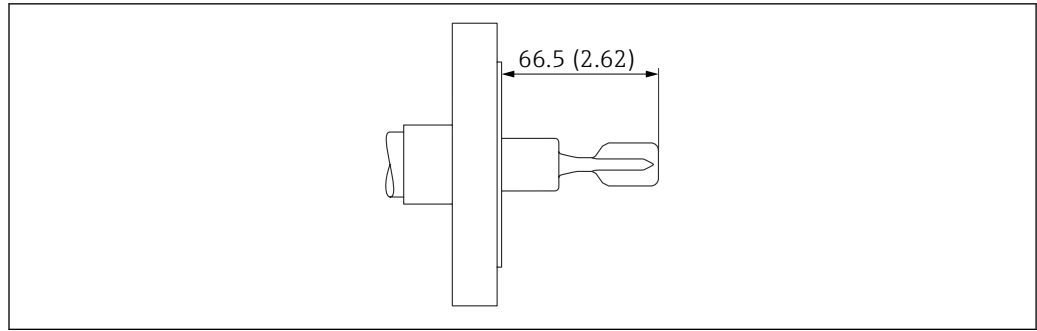
图 54 示意图。测量单位 mm (in)
