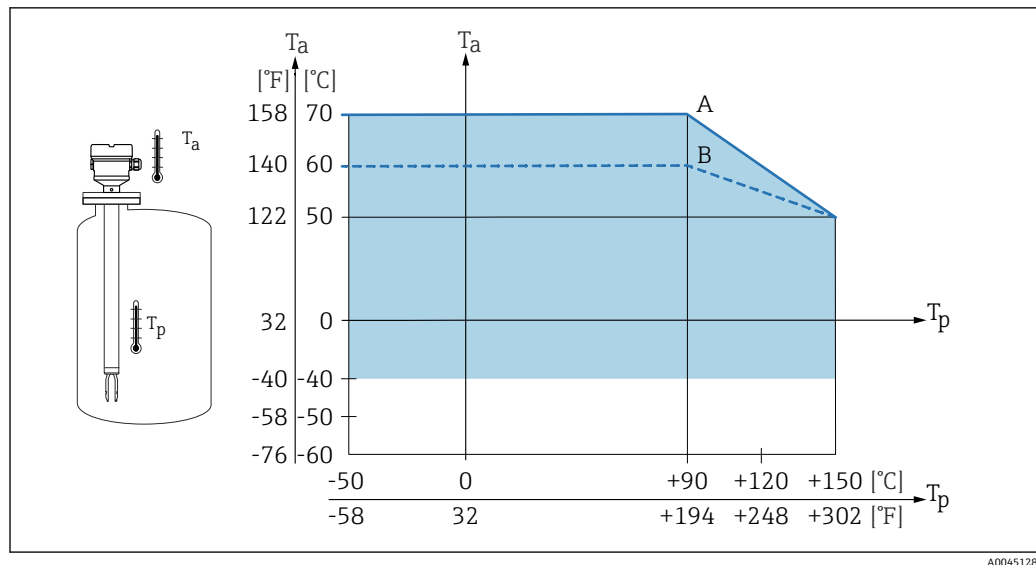
图 31 外壳允许环境温度 T_a 与容器内部过程温度 T_p 的关系：
