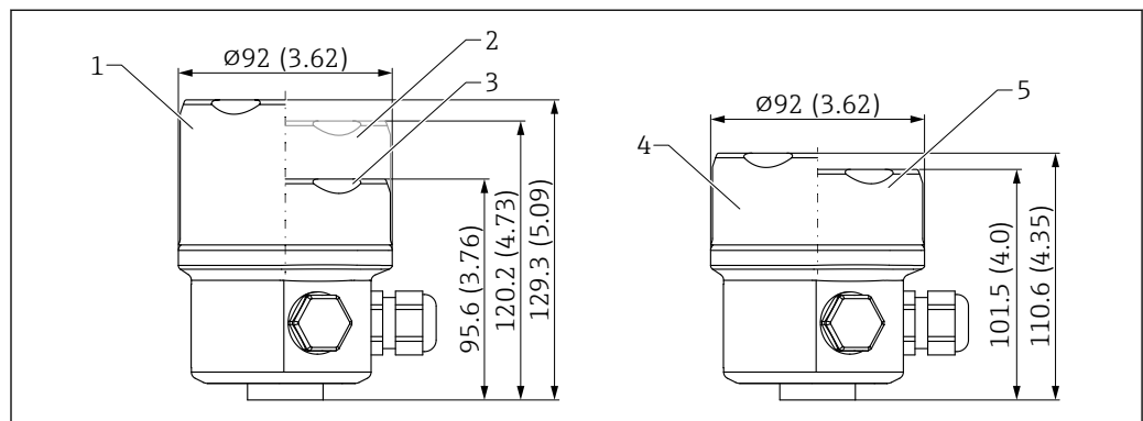
图 37 单腔室 316L 外壳（卫生型）的外形尺寸示意图。测量单位 mm (in)
