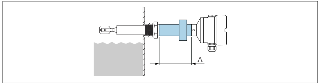
图 39 隔爆玻璃馈通（搭配延长管使用）
