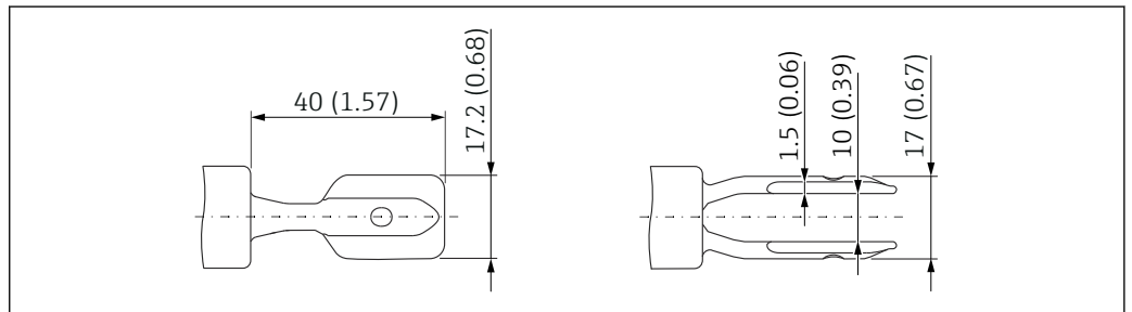
图 42 叉体。测量单位 mm (in)
