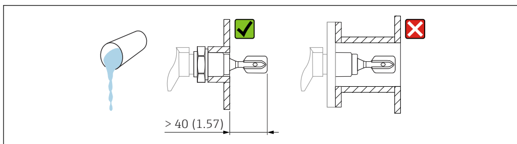
图 21 安装实例：测量高粘度液体。测量单位 mm (in)
