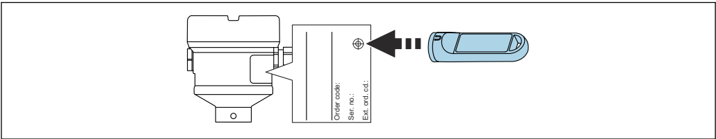
58 使用测试磁铁进行功能测试
