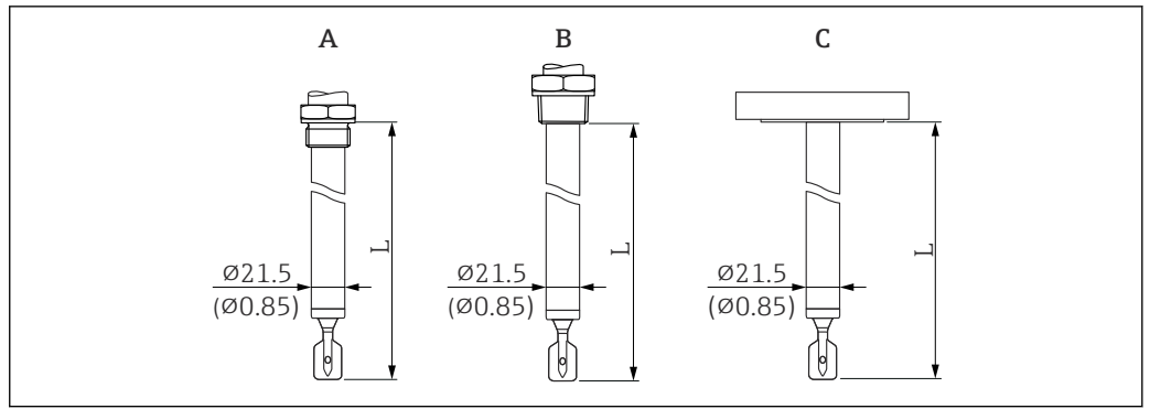
图 41 探头类型：延长管型、短管型（传感器长度 L）。测量单位 mm (in)
