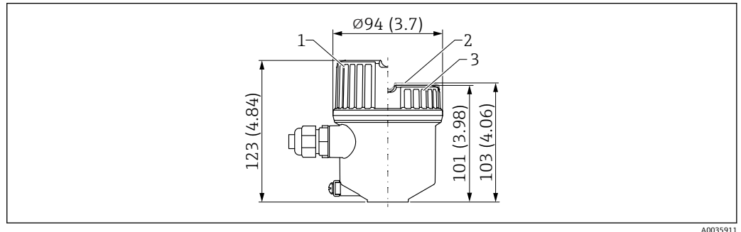
图 33 单腔体塑料外壳的外形尺寸示意图。测量单位 mm (in)
