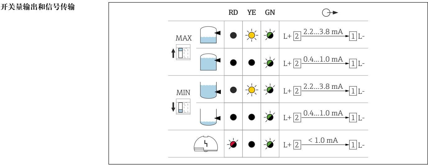
图 14 电子插件 FEL68 的开关量输出和信号传输 MAXDIP 开关：高限（MAX）检测 MIN DIP 开关：低限（MIN）检测 RD 红色 LED 指示灯：报警 YE 黄色 LED 指示灯：开关状态 GN 绿色 LED 指示灯：设备工作状态
