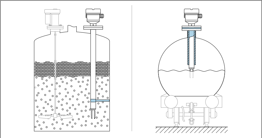
图 29 实例：存在动态负载时，应支撑设备
