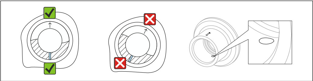
图 30 焊座，带泄漏检测孔
