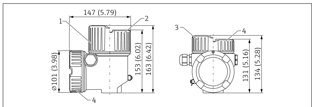
图 38 双腔体 L 型铝外壳（带涂层）的外形尺寸示意图；Ex d/XP、粉尘防爆场合。测量单位 mm (in)
