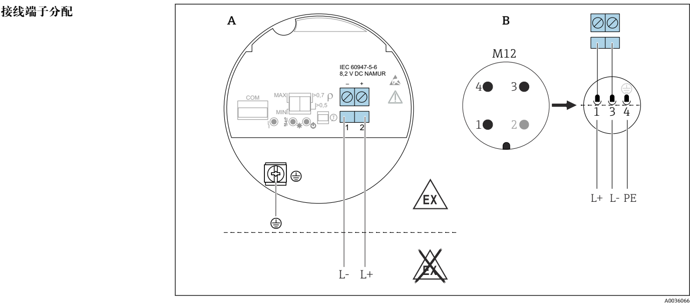
图 13 电子插件 FEL68：两线制连接，NAMUR 信号（≥ 2.2 mA / ≤ 1.0 mA） A 使用接线端子接线 B 根据 EN61131-2 标准，使用外壳中的 M12 插头接线
