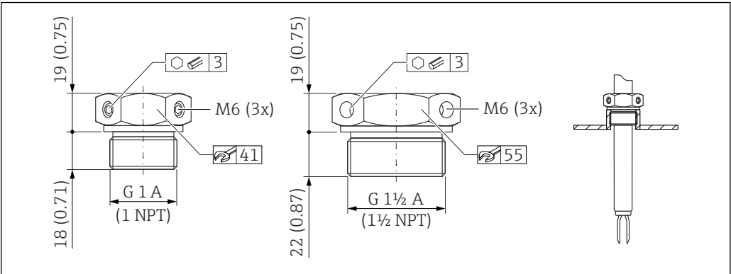
66 常压滑动套管 p_e = 0 \text{ bar (0 psi)} 。测量单位 mm (in)
