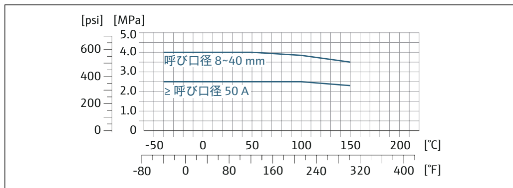
図 13 接続部の材質 1.4404 (SUS 316 相当または SUS 316L 相当)
