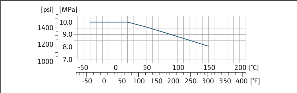
図 16 接続部の材質 1.4404 (SUS 316 相当または SUS 316L 相当)
