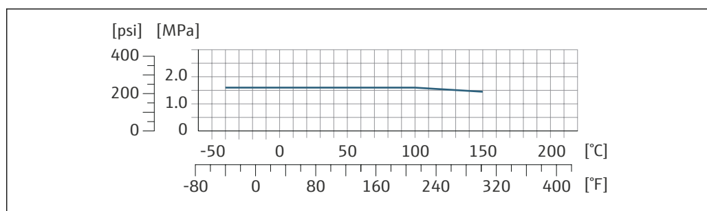
図 14 接続部の材質 1.4404 (SUS 316 相当または SUS 316L 相当)
