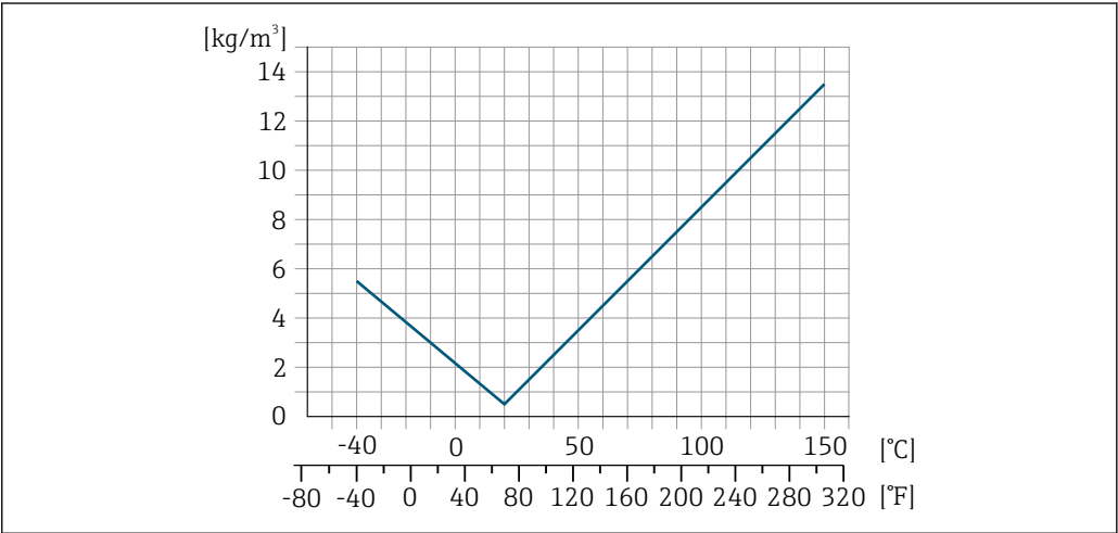
図 5 現場密度調整、例：+20 °C (+68 °F) 時
