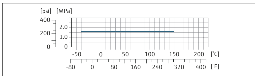
図 15 接続部の材質 1.4404 (SUS 316 相当または SUS 316L 相当)
