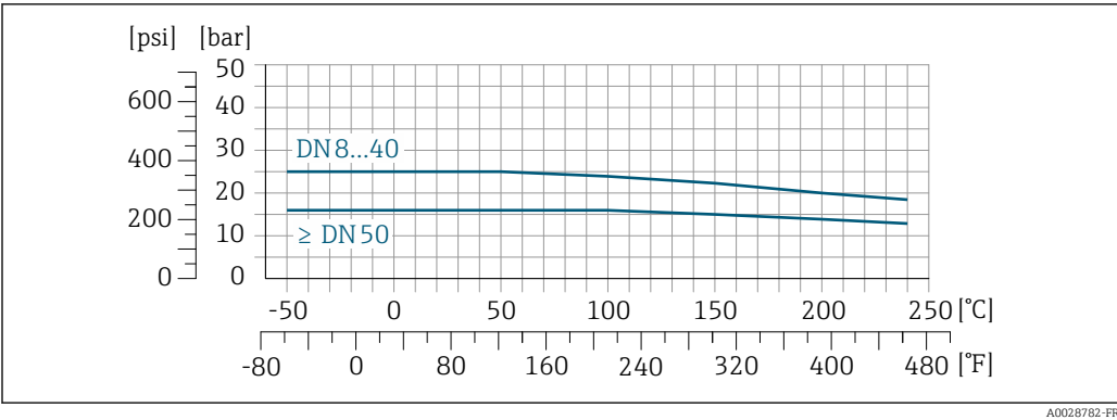
20 Avec matériau de raccord 1.4404 (316/316L)
