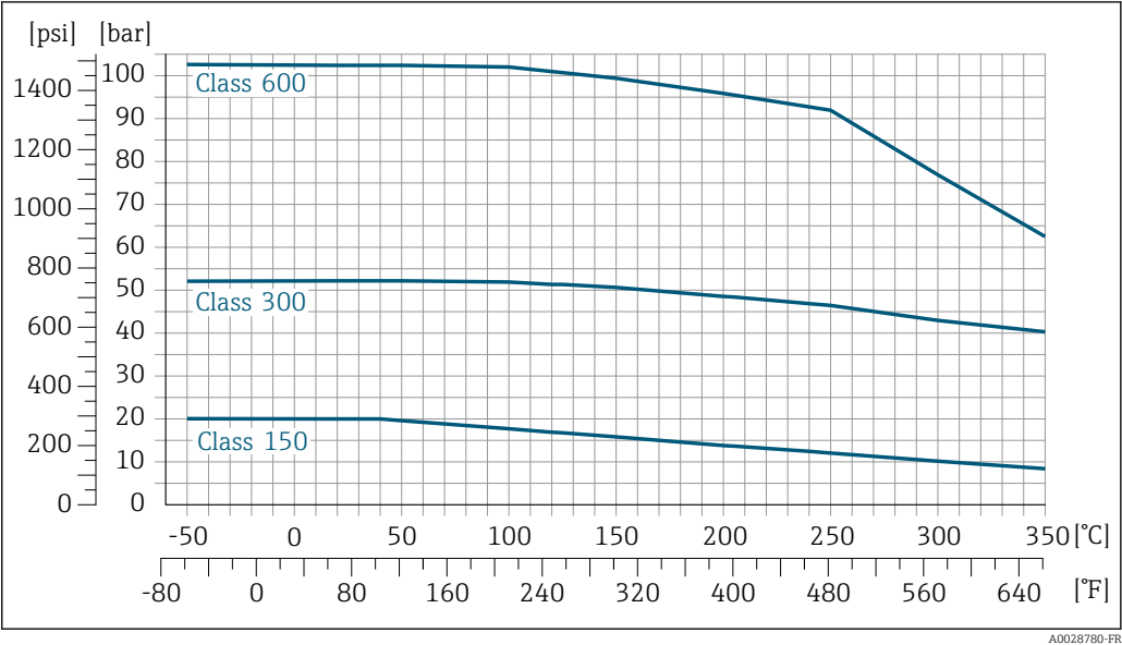
18 Avec matériau de bride Alloy C22
