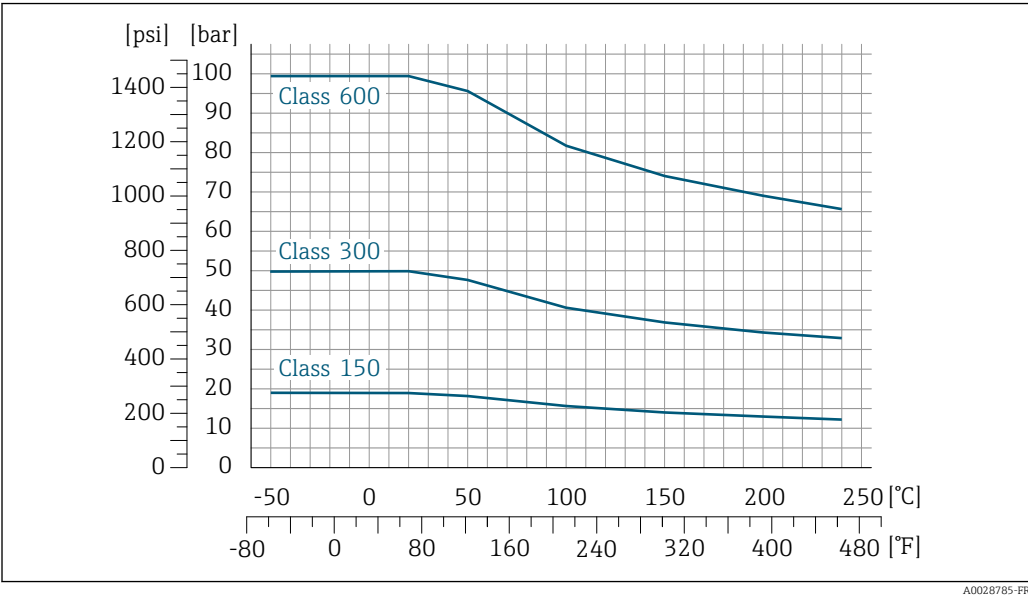
22 Avec matériau de bride 1.4301 (F304) ; pièces en contact avec le produit Alloy C22
