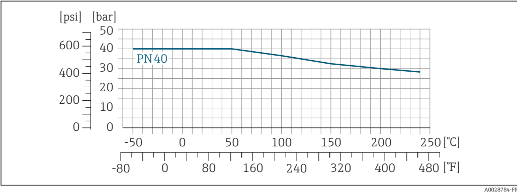
21 Avec matériau de bride 1.4301 (F304) ; pièces en contact avec le produit Alloy C22
