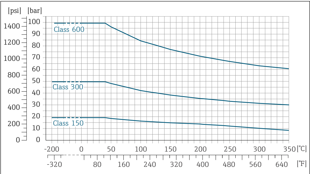
17 Avec matériau de bride 1.4404 (F316/F316L)
