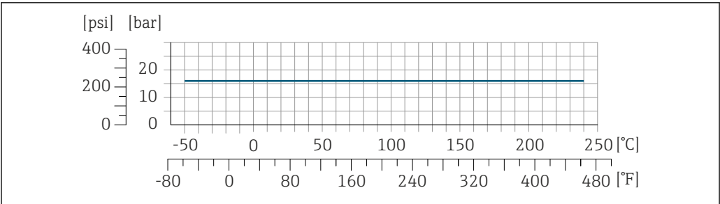
27 Avec matériau de raccord 1.4404 (316/316L)
