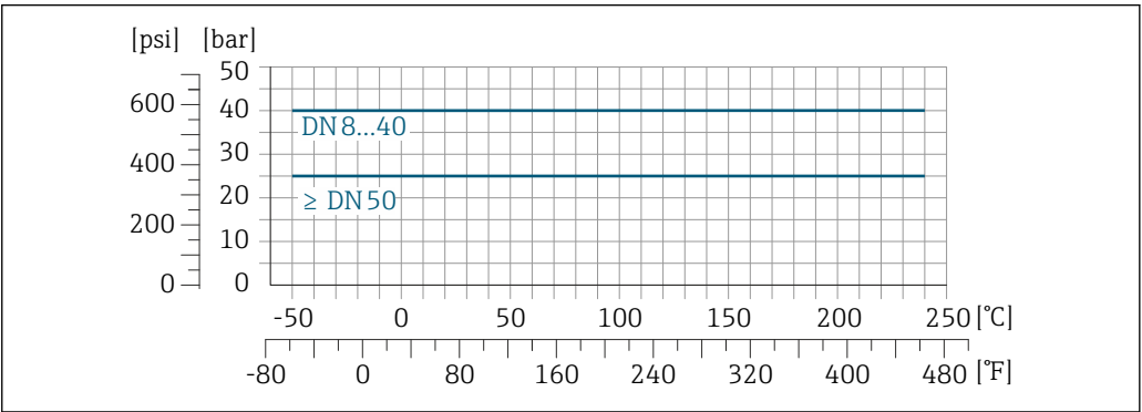
25 Avec matériau de raccord 1.4404 (316/316L)
