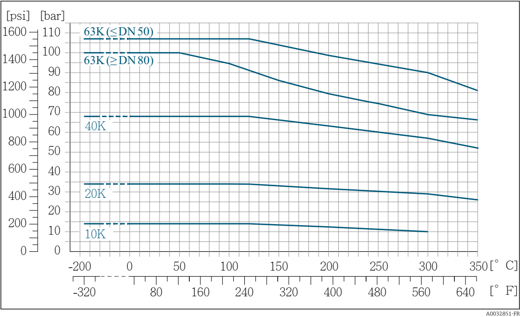
19 Avec matériau de bride 1.4404 (F316/F316L), Alloy C22
