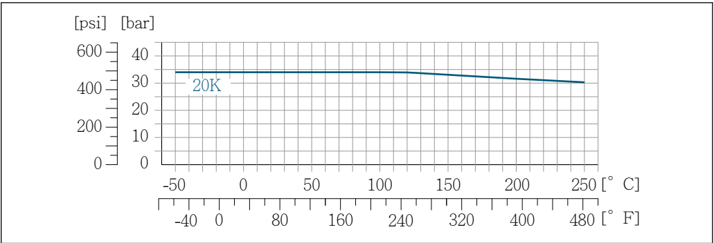
23 Avec matériau de bride 1.4301 (F304) ; pièces en contact avec le produit Alloy C22
