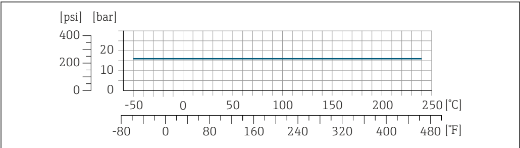
26 Avec matériau de raccord 1.4404 (316/316L)
