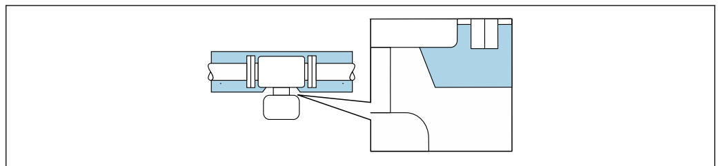
29 Isolation thermique avec tube prolongateur exposé
