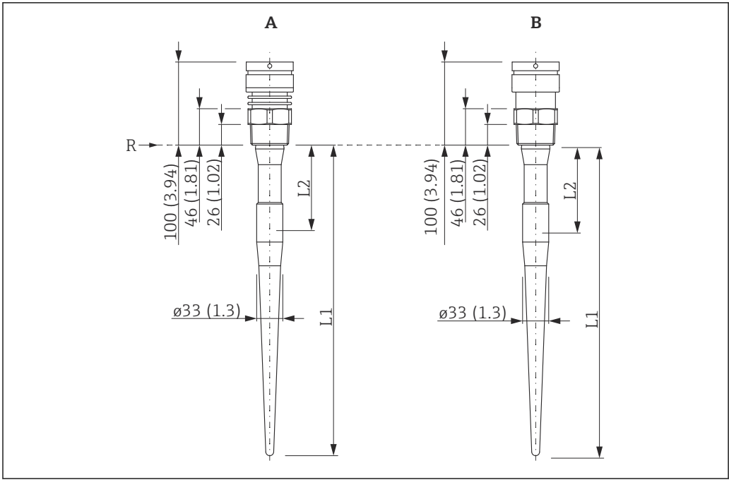
28 Размеры прибора с резьбой. Единица измерения мм (дюйм)
