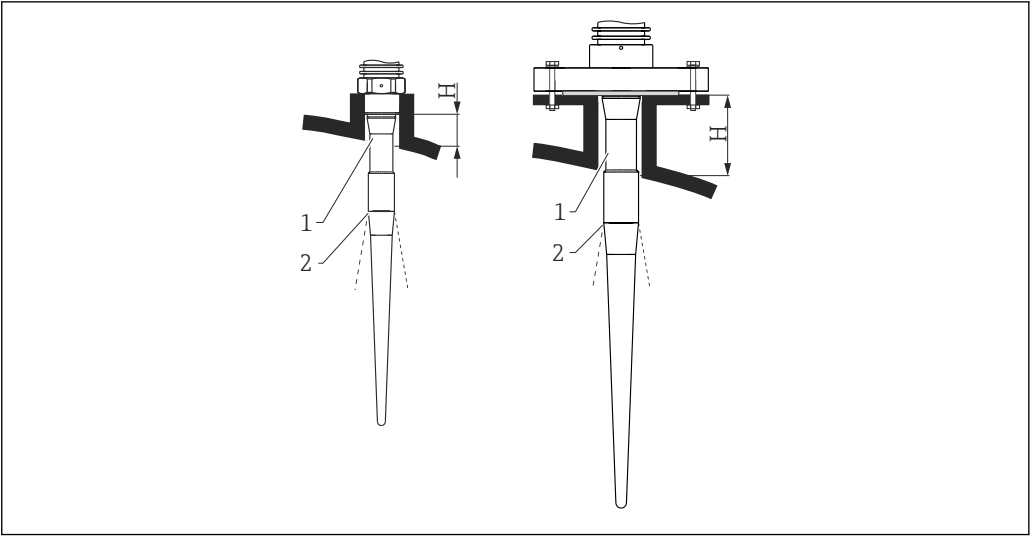
19 Высота штуцера для стержневой антенны (FMR53)
