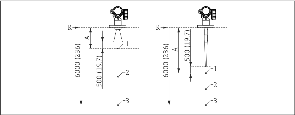
40 Точки калибровочного протокола по 3 точкам; единица измерения: мм (дюймы)
