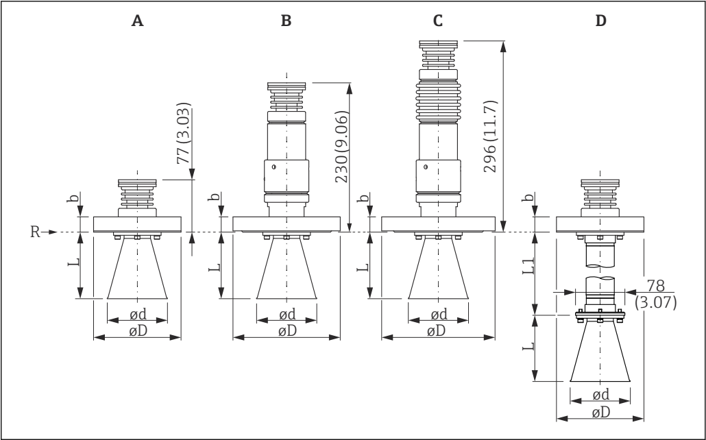
29 Размеры прибора FMR54 с рупорной антенной. Единица измерения мм (дюйм)
