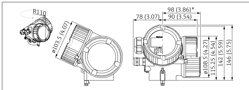
■ 24 Корпус GT18 (316L). Единица измерения мм (дюйм)
