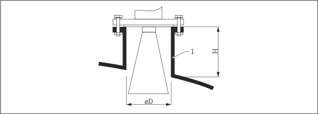
20 Высота и диаметр штуцера для рупорной антенны
