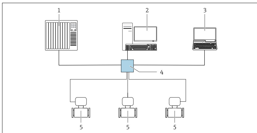
40 Options de configuration à distance via Modbus TCP sur Ethernet - 100 Mbit/s : topologie en étoile
