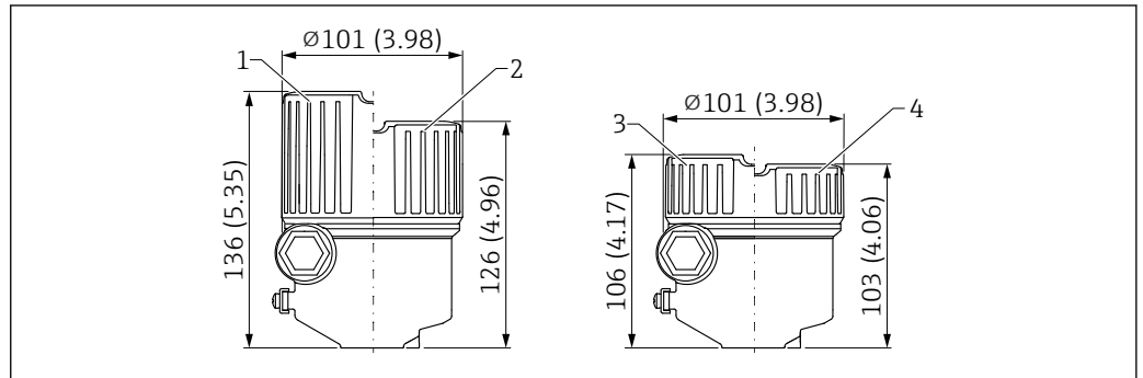
35 Medidas de la caja de compartimento único, aluminio, recubierta. Unidad de medida mm (in)
