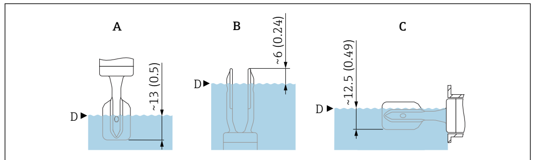
17 Puntos de conmutación típicos, horquilla vibratoria recubierta de plástico (ECTFE, PFA), medidas sin el grosor del recubrimiento. Unidad de medida mm (in)
