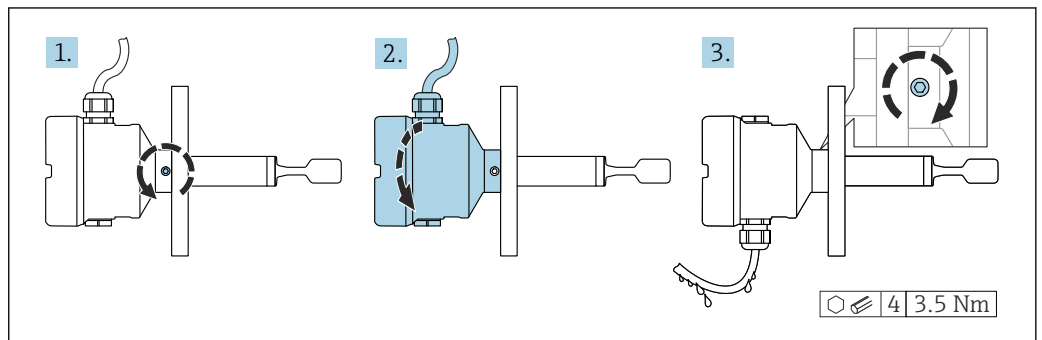
29 Caja con tornillo de bloqueo externo y circuito de goteo
