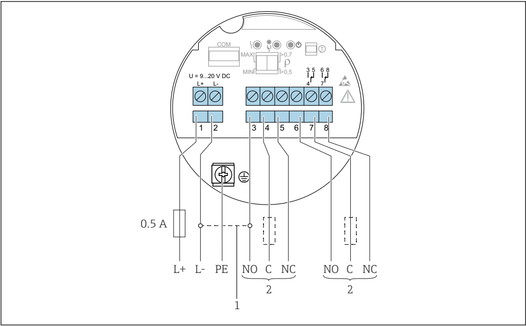
9 Conexión CC con salida de relé, módulo del sistema electrónico FEL64 DC 1 Cuando está puenteada, la salida de relé trabaja con lógica NPN 2 Carga conectable
