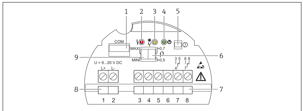
45 Ejemplo de módulo de la electrónica FEL64DC
