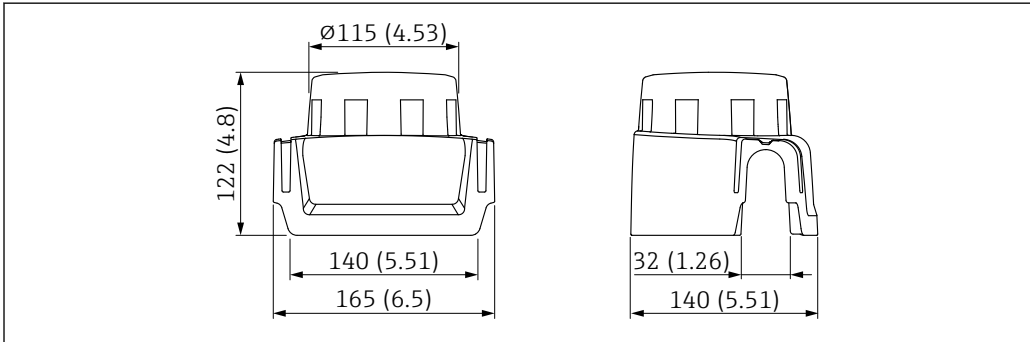
53 Medidas de la cubierta protectora, plástico, XW111. Unidad de medida mm (in)
