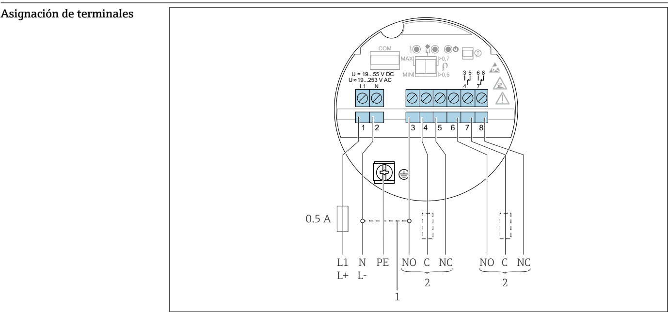
7 Conexión universal de corriente con salida de relé, módulo de la electrónica FEL64
