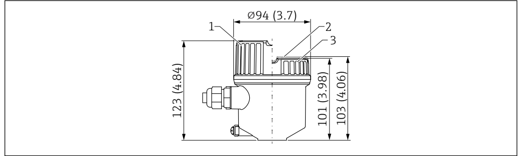
34 Medidas de la caja de compartimento único, plástico. Unidad de medida mm (in)
