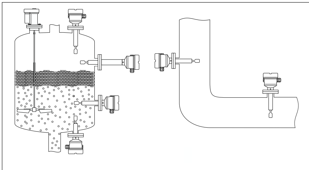
21 Ejemplos de instalación para un depósito, tanque o tubería
