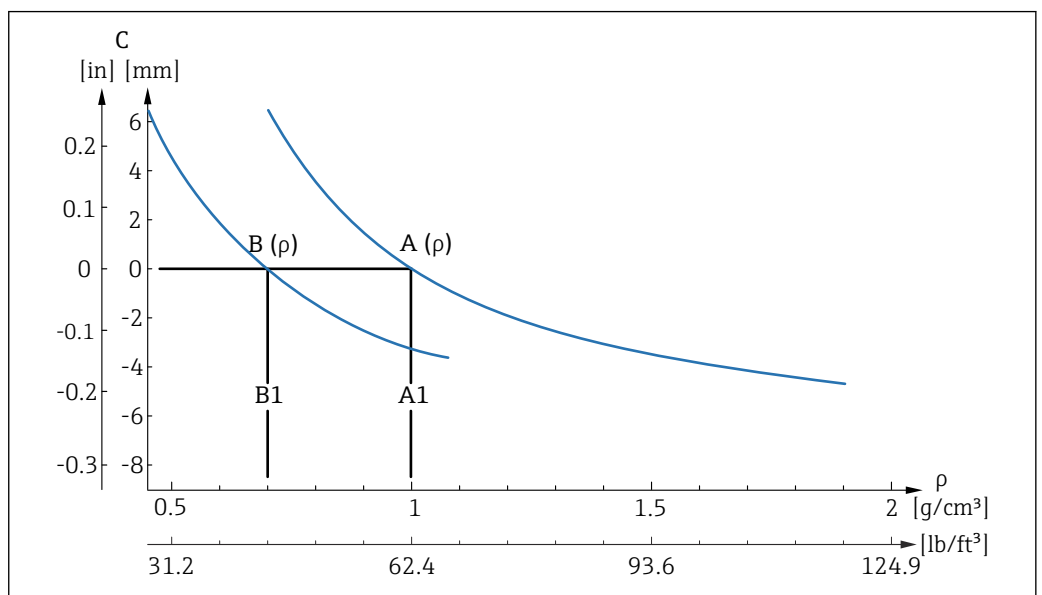
20 Puntos de conmutación de referencia a partir de la densidad, recubrimiento de esmalte
