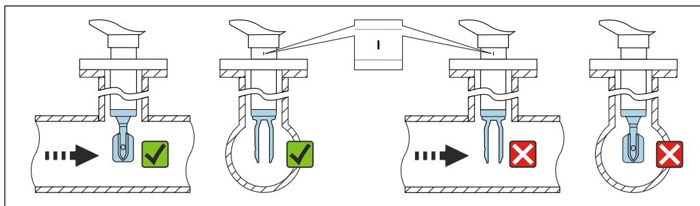
27 Instalación en tuberías (tenga en cuenta la posición de la horquilla y las marcas)
