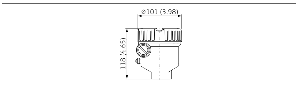
37 Medidas de la caja de compartimento único de 316L; también con Ex d/XP, a prueba de ignición por polvo; cubierta sin mirilla. Unidad de medida mm (in)
