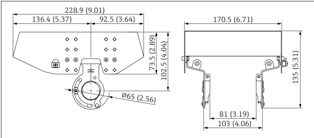
52 Medidas de la cubierta protectora, 316 L, XW112. Unidad de medida mm (in)
