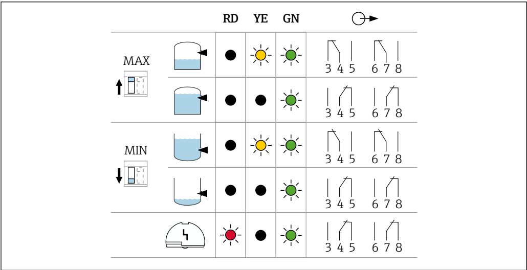
10 Comportamiento de la salida de conmutación y de la señalización, módulo del sistema electrónico FEL64 DC
