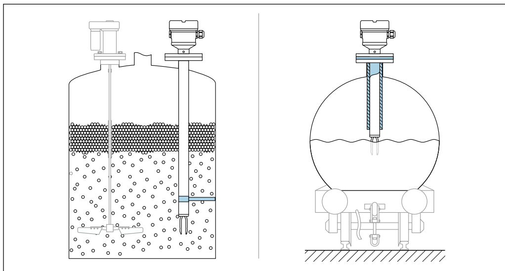
31 Ejemplos de soporte en caso de carga dinámica
