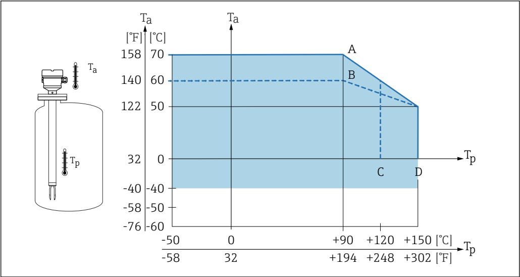
32 Temperatura ambiente admisible T_a en la caja en función de la temperatura de proceso T_p en el depósito:
