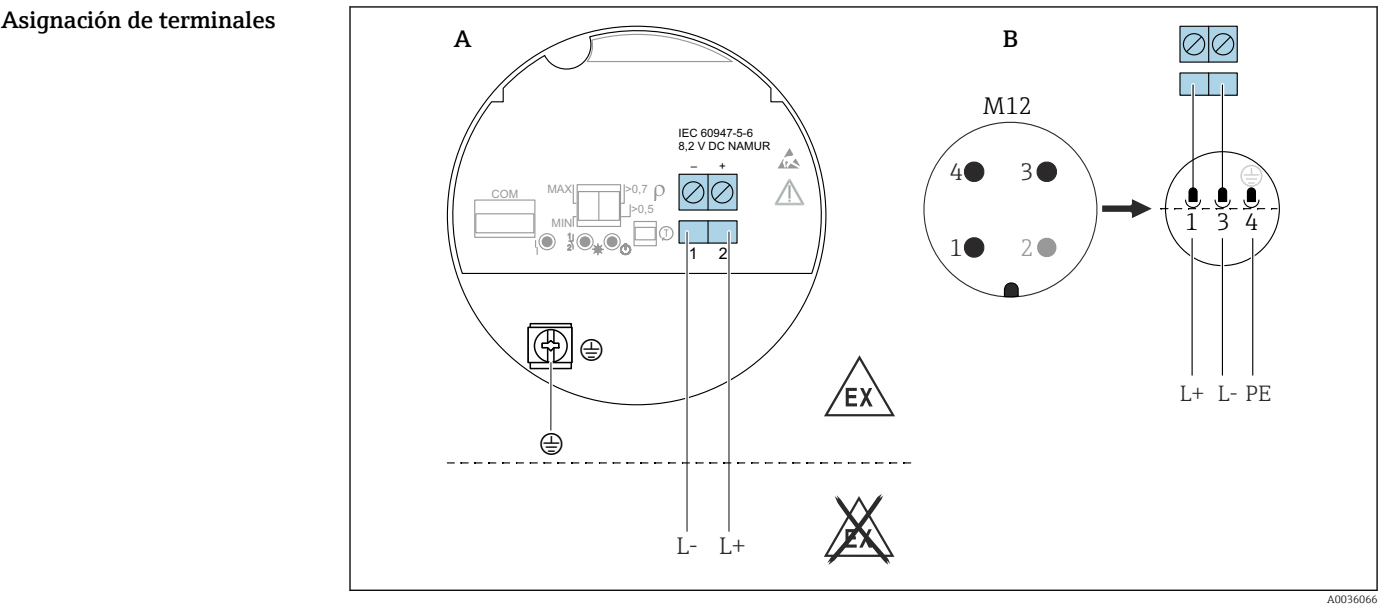
13 NAMUR a 2 hilos \geq 2,2 \text{ mA} / \leq 1,0 \text{ mA} , módulo del sistema electrónico FEL68
