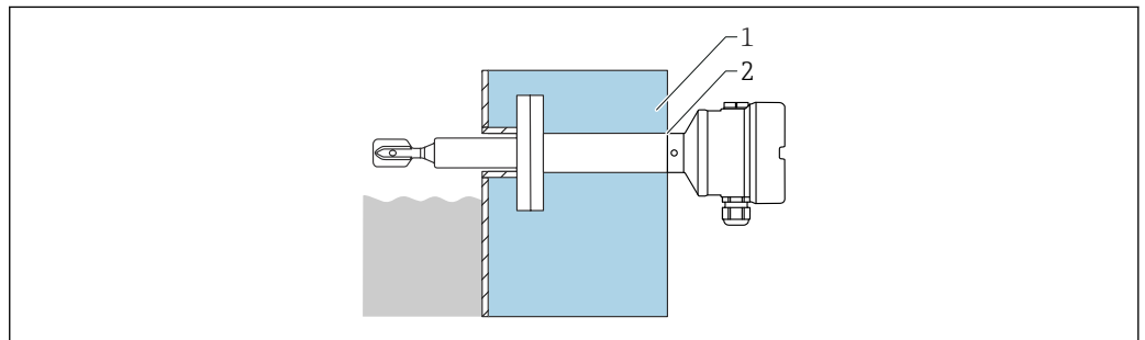
30 Depósito con aislamiento contra el calor (ejemplo con distanciador de temperatura)
