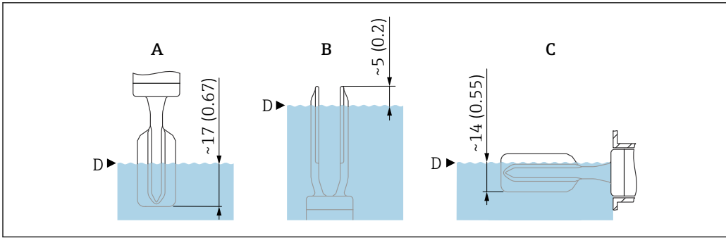
18 Puntos de conmutación típicos, horquilla vibratoria recubierta de esmalte, medidas sin el grosor del recubrimiento. Unidad de medida mm (in)
