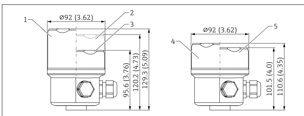
38 Medidas de la caja de compartimento único, 316L, higiénica. Unidad de medida mm (in)
