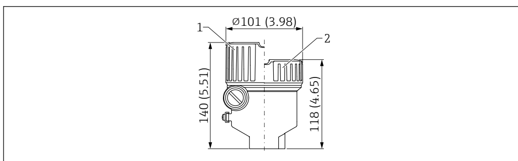
36 Medidas de la caja de compartimento único, aluminio, recubierto; con Ex d/XP, a prueba de ignición por polvo. Unidad de medida mm (in)
