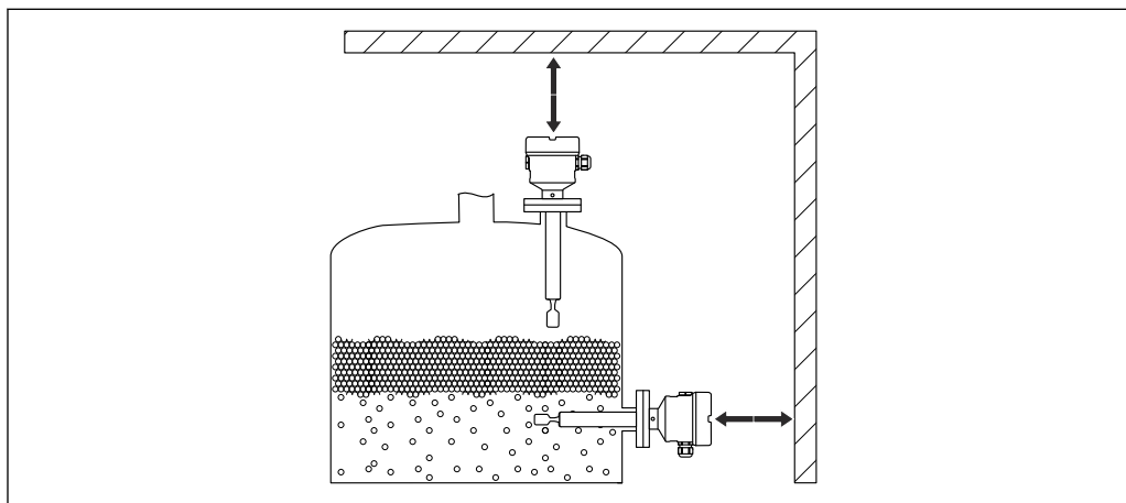
25 Tenga en cuenta el espacio expedito
