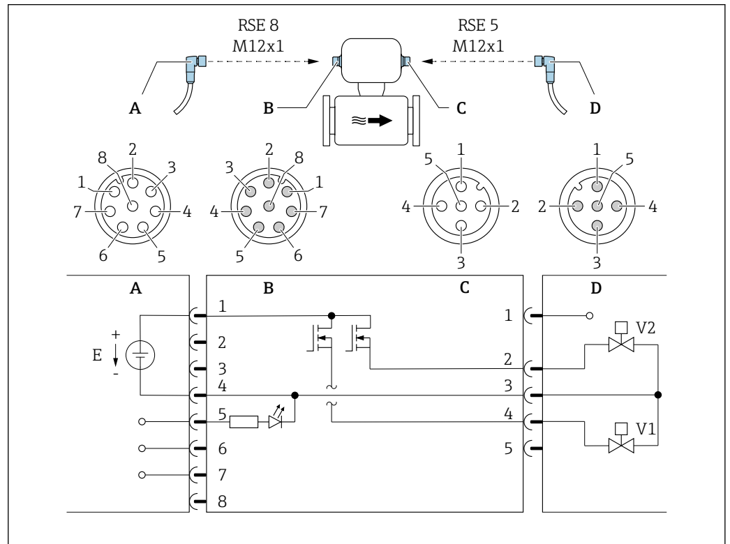
图 6 连接仪表
