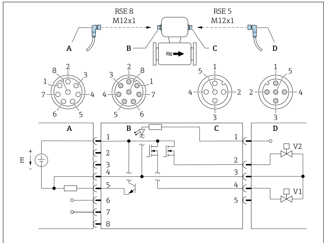
图 7 连接仪表
