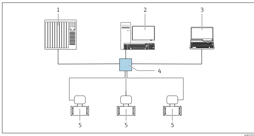
58 Opções para operação remota através do Modbus TCP por Ethernet - 100 Mbit/s: Topologia estrela
