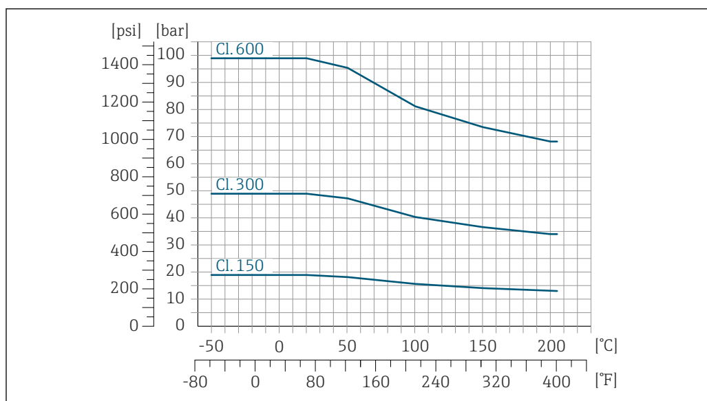
26 Flange da junta de lapela com material do flange: 1.4301 (F304), partes úmidas Liga C22: 2.4602 (UNS N06022)
