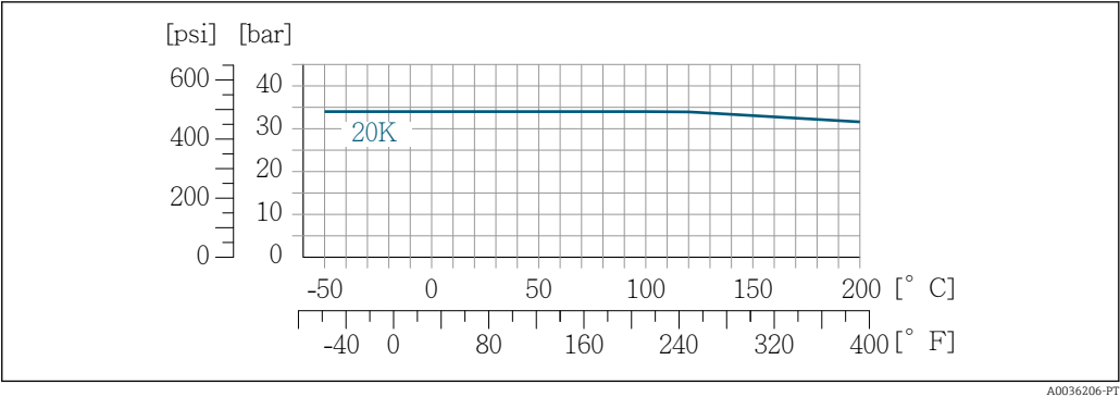
28 Flange da junta de lapela com material do flange: 1.4301 (F304), partes úmidas Liga C22: 2.4602 (UNS N06022)
