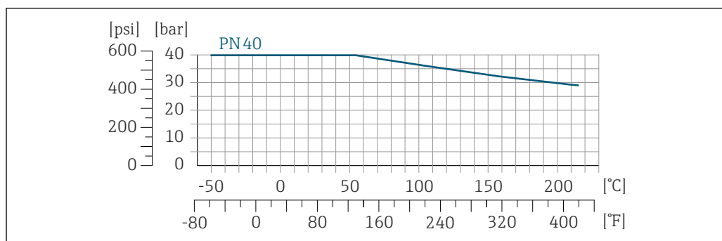
23 Flange da junta de lapela com material do flange: 1.4301 (F304), partes úmidas Liga C22: 2.4602 (UNS N06022)
