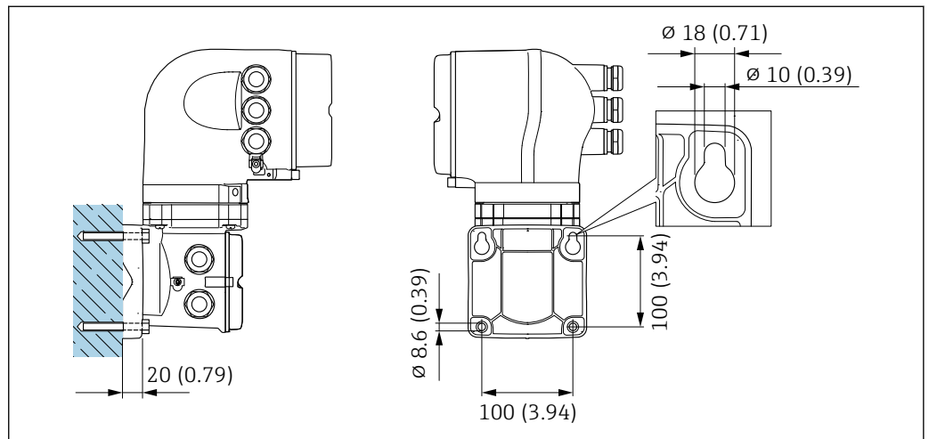
17 Unidade em mm (pol.)
