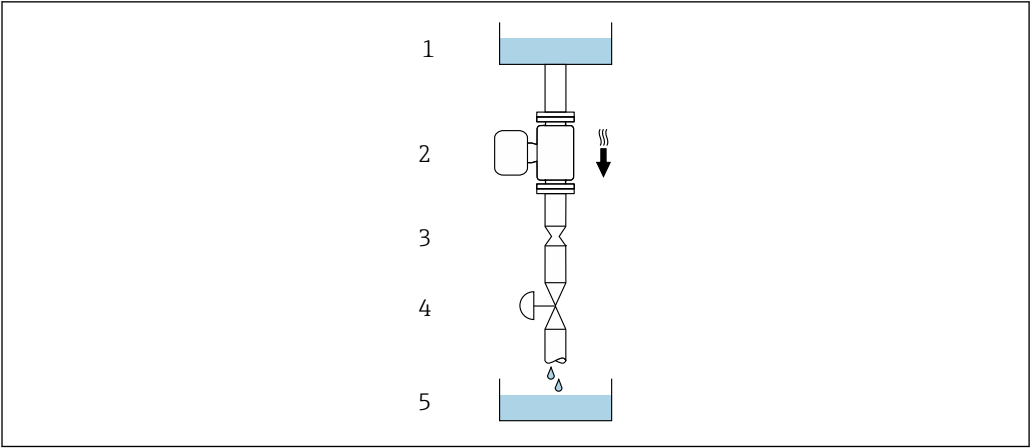
13 Instalação em um tudo descendente (por exemplo para aplicações de batelada)
