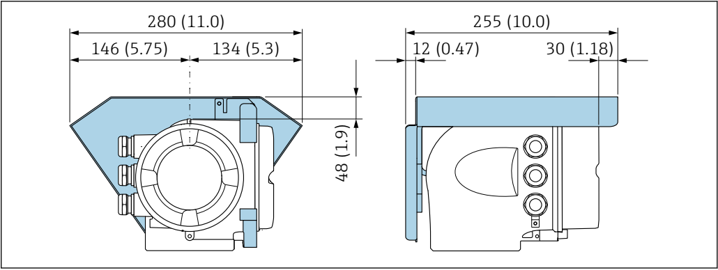
19 Tampa de proteção contra tempo para Proline 500 - unidade mm (pol.)
