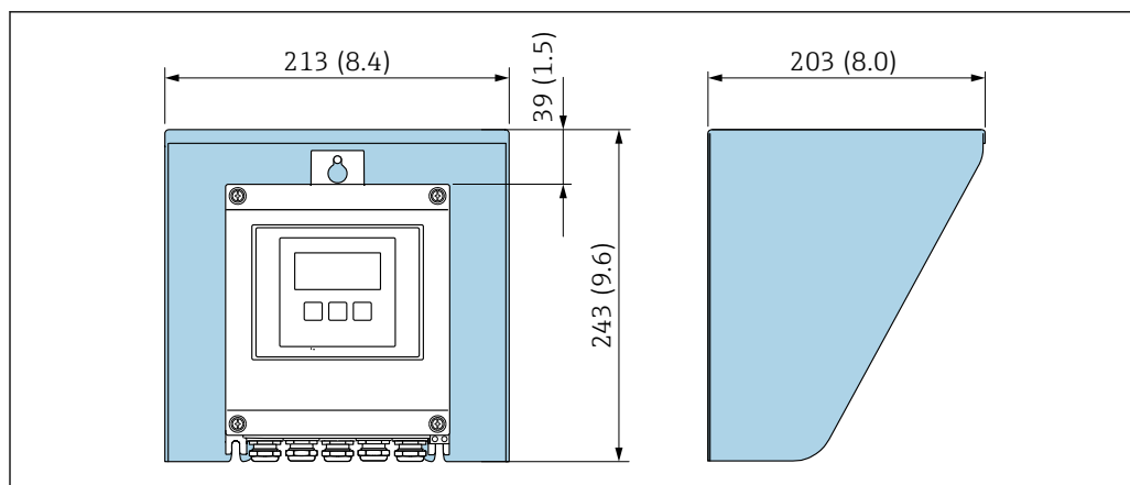
39 Tampa de proteção contra tempo para Proline 500 - digital; unidade mm (pol.)
