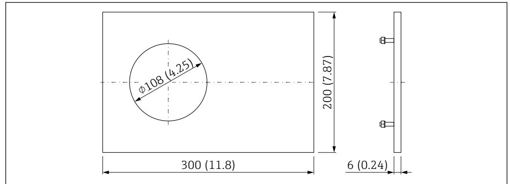
图 20 挡板，1.4301，传感器开孔 \varnothing 108 mm (4.25 in)。测量单位 mm (in)
