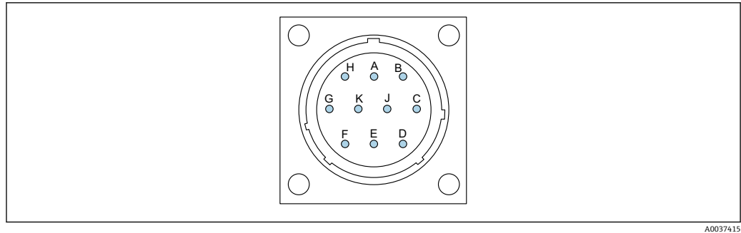
图 12 10 针插头的针脚分配
