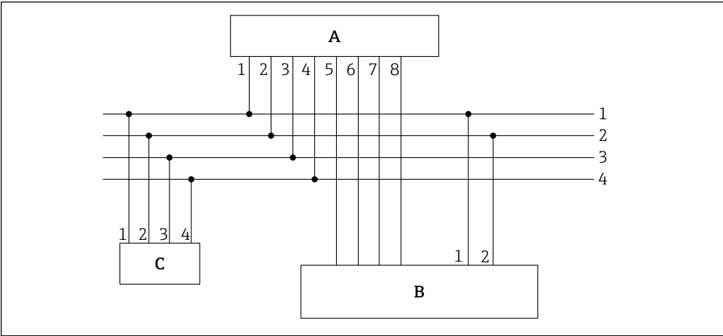
图 16 接线示例：连接电缆的仪表端带 10 针插座，末端线芯上安装有线鼻子
