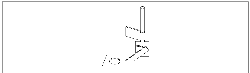
图 21 通用安装支座（1.4301 材质），配备倾转装置和固定头，传感器开孔直径 \varnothing 108 mm (4.25 in)
