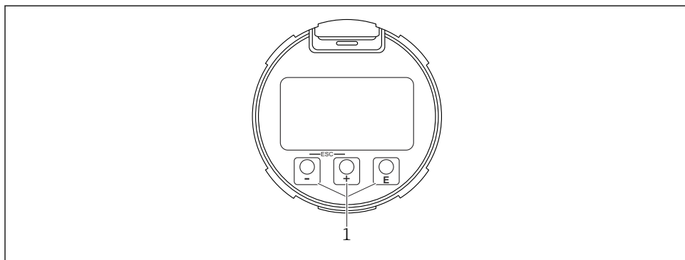
21 Display grafico con tasti operativi ottici (1)
