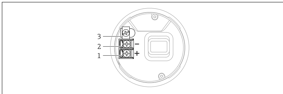
16 Morsetti di connessione e morsetto di terra nel vano connessioni, custodia a vano unico
