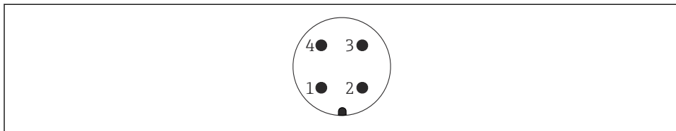
19 Vista della connessione sul dispositivo
