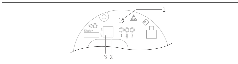
20 Tasto operativo e microinterruttori sull'inserto elettronico (FEL60P) - Ethernet-APL
