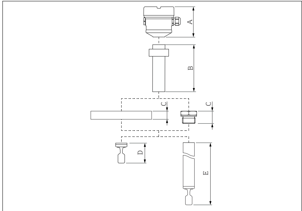
図 30 本体高さを計算するための構成部品
