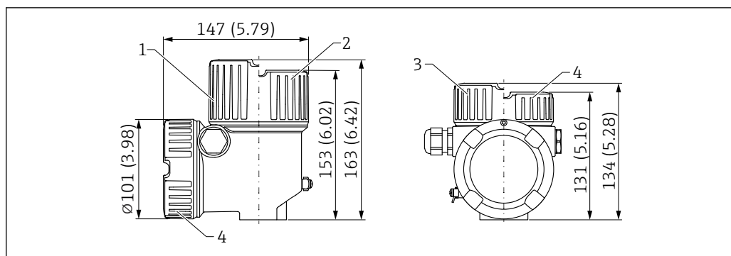
図 36 デュアルコンパートメントハウジング、L字型、アルミニウム、コーティングの寸法 (Ex d/XP、粉塵防爆仕様)。測定単位 mm (in)
