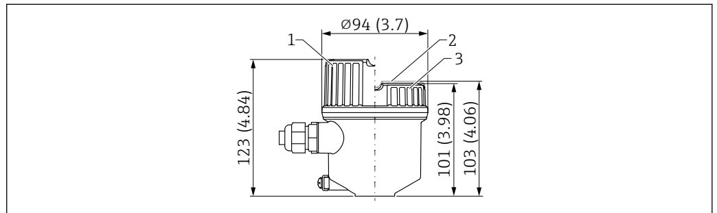
図 31 シングルコンパートメントハウジング、プラスチックの寸法。測定単位 mm (in)
