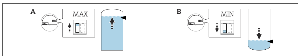
図 50 上限 (MAX) /下限 (MIN) のエレクトロニクインサートのスイッチ位置
