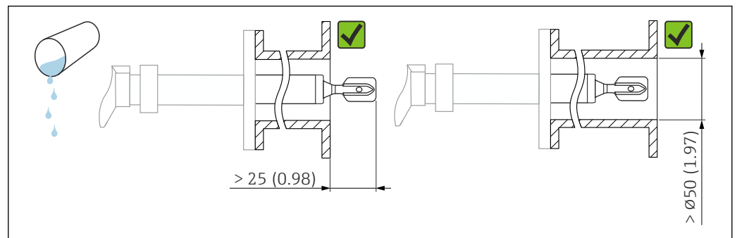
図 19 低粘度液体の設置例。測定単位 mm (in)
