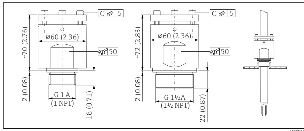
図 61 高圧用スライディングスリーブ。測定単位 mm (in)
