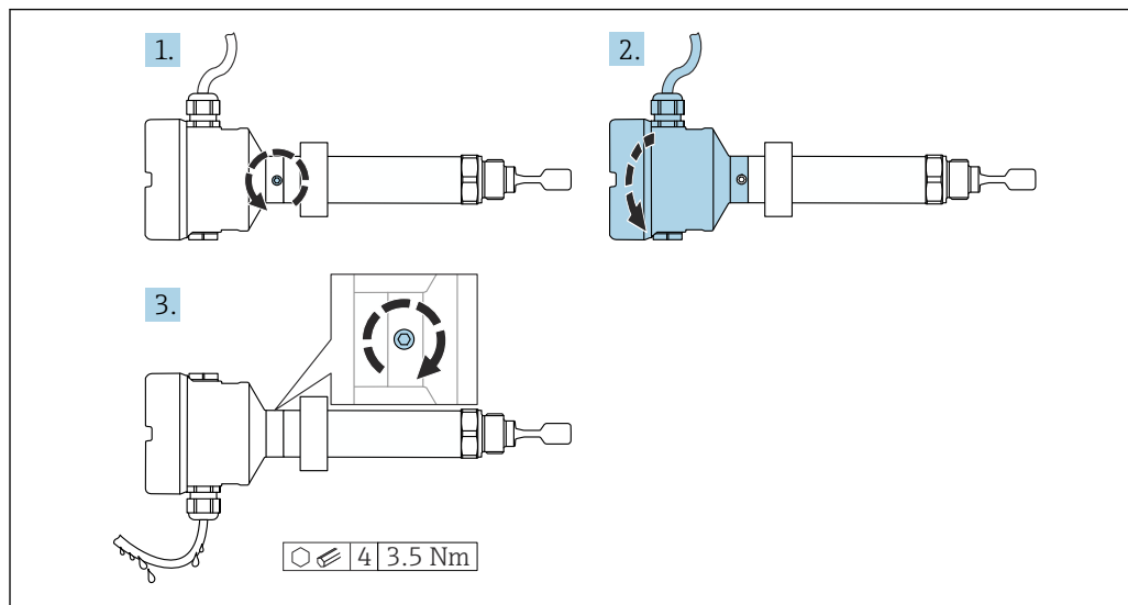
図 26 外部のロックネジおよびドリッブループ付きハウジング
