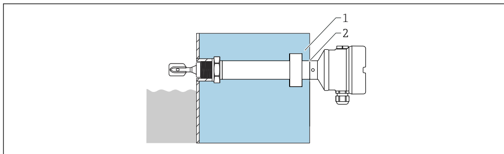
図 27 断熱材付きタンクへの設置
