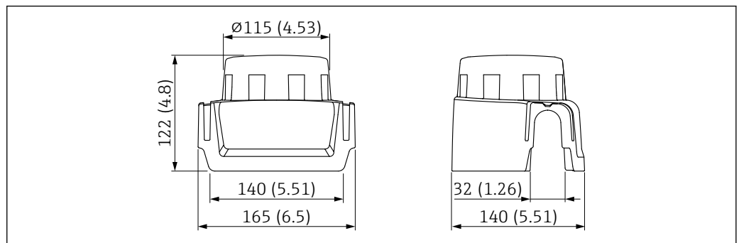
図 57 保護カバー、プラスチック、XW111 の寸法。測定単位 mm (in)
