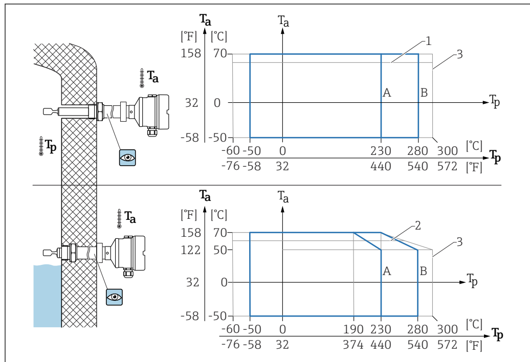
図 29 ハウジングの許容周囲温度 T_a は、容器内のプロセス温度 T_p に応じて異なります。
