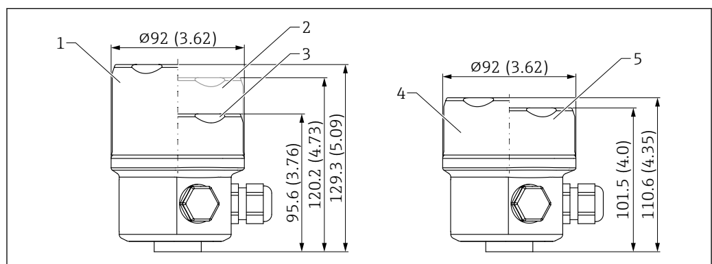
図 35 シングルコンパートメントハウジング、SUS 316L 相当、サニタリ仕様の寸法。測定単位 mm (in)
