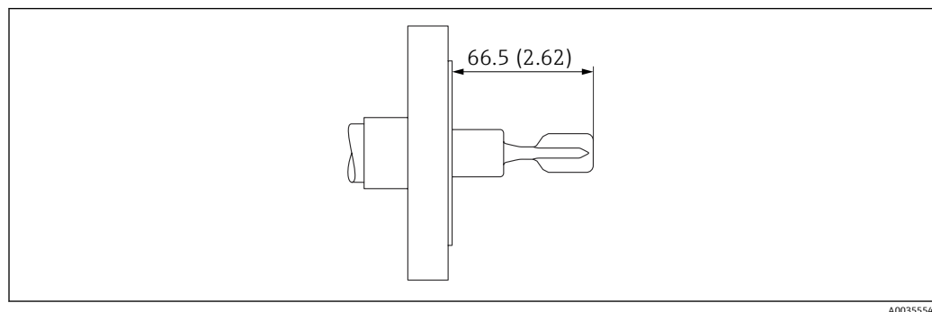
48 サンプル図。測定単位 mm (in)
