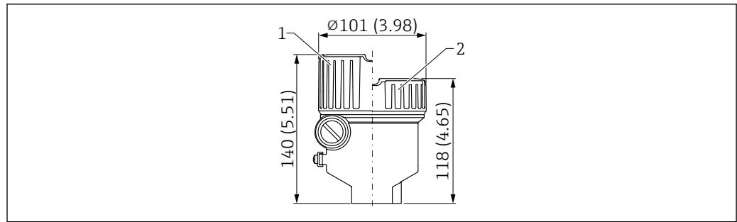
図 33 シングルコンパートメントハウジング、アルミニウム、コーティングの寸法（Ex d/XP、粉塵防爆仕様）。測定単位 mm (in)
