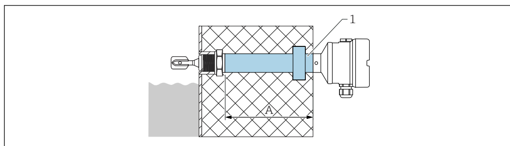
図 37 ガラスガスタイトフィードスルー付き温度セパレータ
