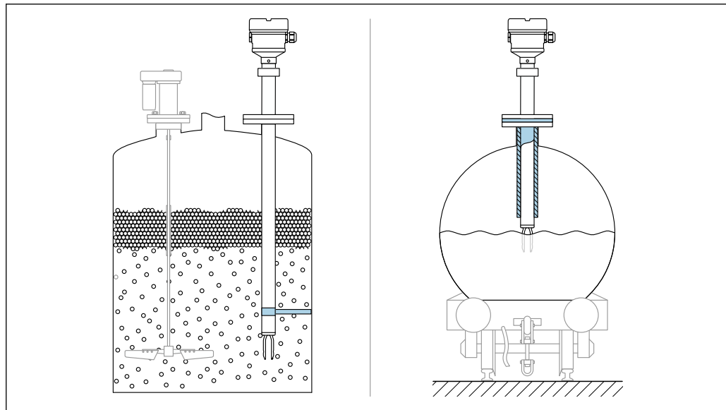
図 28 動的負荷が発生する場合のサポートの例
