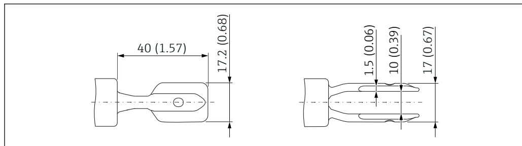
図 40 音叉部。測定単位 mm (in)
