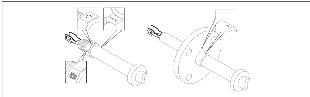
図 23 マークを使用して容器に水平に設置する場合の音叉部の位置
