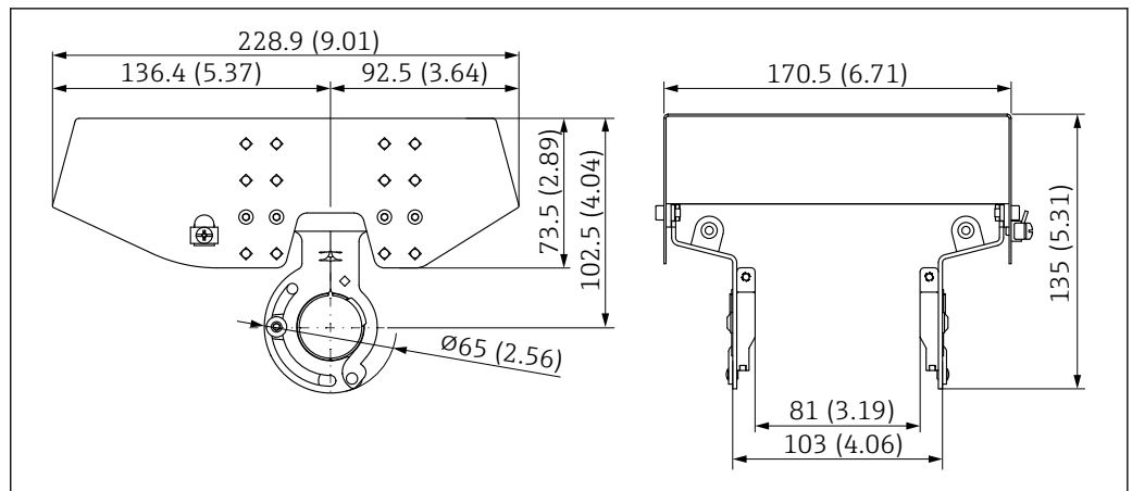
図 56 保護カバー、SUS 316L 相当、XW112 の寸法。測定単位 mm (in)
