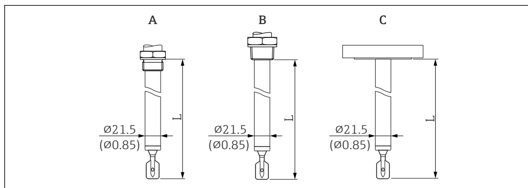
図 39 伸長パイプ (センサ長 L)。測定単位 mm (in)
