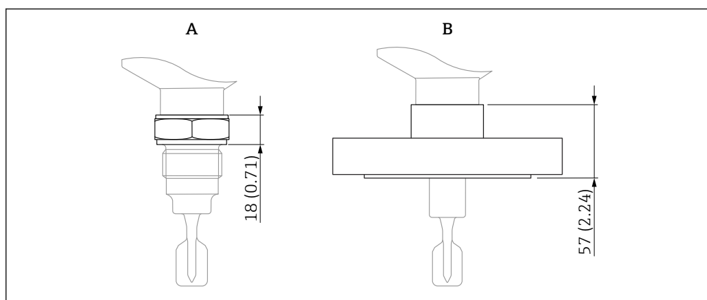
図 41 プロセス接続の最大高さ仕様
