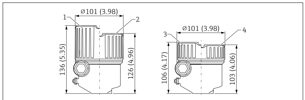
図 32 シングルコンパートメントハウジング、アルミニウム、コーティングの寸法。測定単位 mm (in)
