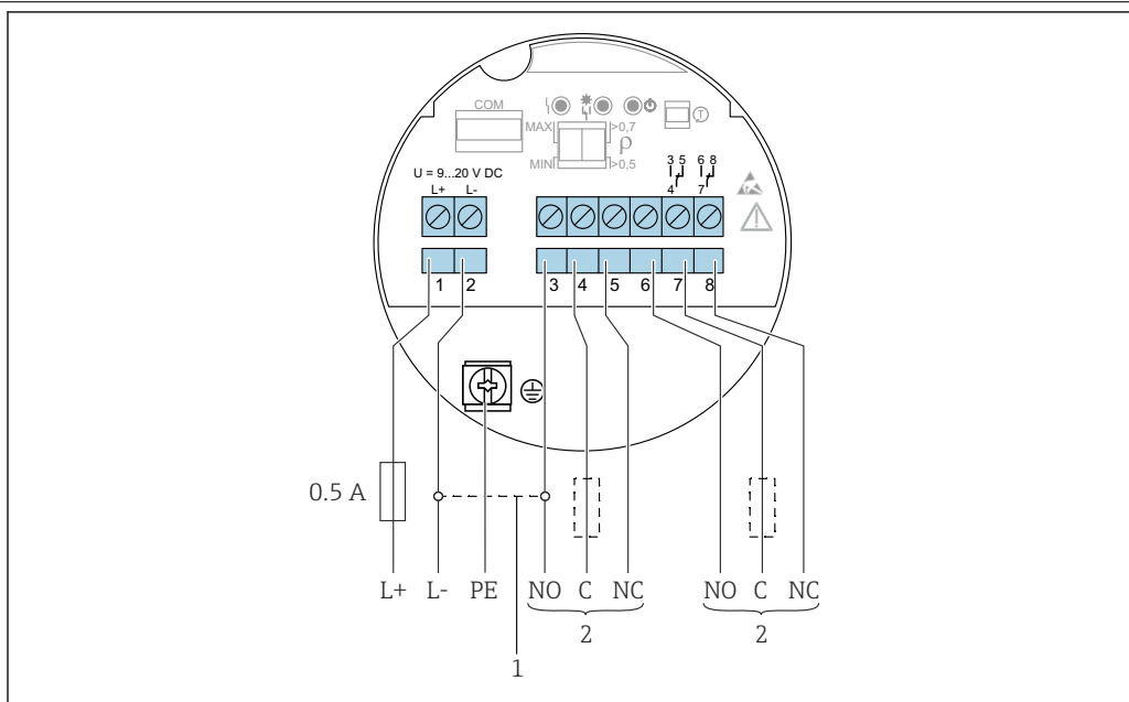
図 9 DC 接続、リレー出力付き、エレクトロニックインサート FEL64 DC
