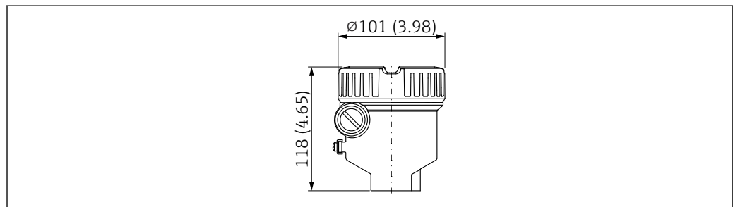
図 34 シングルコンパートメントハウジング、SUS 316L 相当の寸法（Ex d/XP および 粉塵防爆仕様、ハウジングカバーの窓なし）。測定単位 mm (in)
