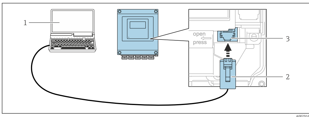
30 Подключение через сервисный интерфейс (CDI-RJ45)
