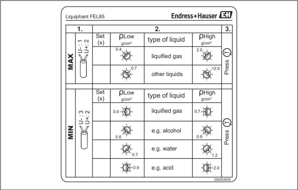
21 Figura: pase del sensor
