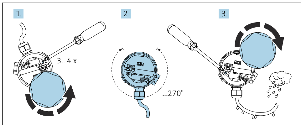
14 Caja con tornillo de bloqueo; forme un circuito de goteo en el cable
