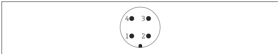
16 Conector M12, asignación de pines
