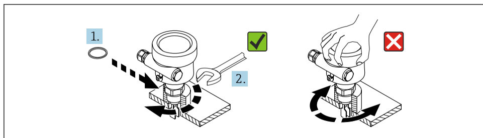
13 Enroscado del equipo
