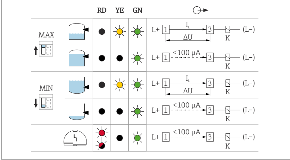
17 Sivî çıkışının davranışı ve sinyaller, elektronik devre FEL62
