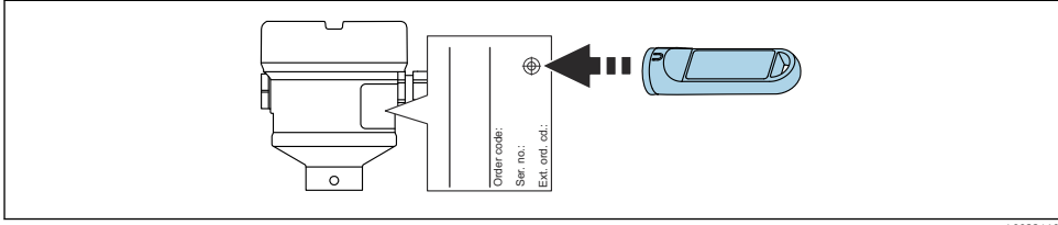
30 Test mıknatısı ile fonksiyon testi
