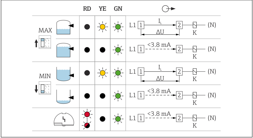
14 Sıvı çıkışının davranışı ve sinyaller, elektronik devre FEL61
