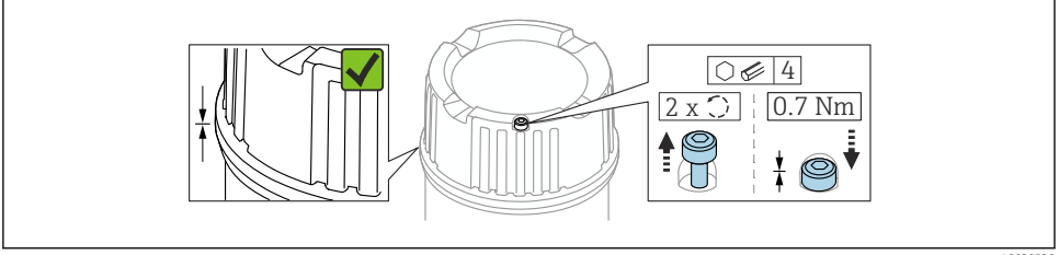
12 Sabitleme vidasına sahip kapak
