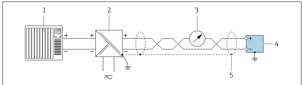
图 25 接线实例：4 ... 20 mA HART 电流输出（无源）
