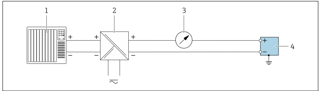
☑ 18 接线实例：4 ... 20 mA 电流输出（无源）
