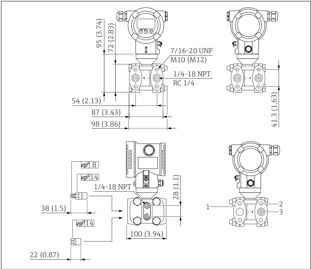
8 Vista frontale, vista lato sinistro e vista lato destro. I dadi si trovano sempre sul lato negativo. Unità di misura mm (in)
