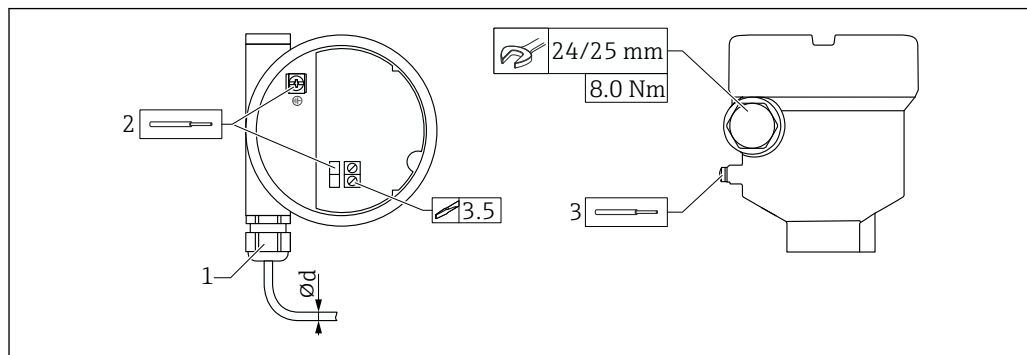
図 20 カップリングの例 (電線口、エレクトロニックインサートと端子)
