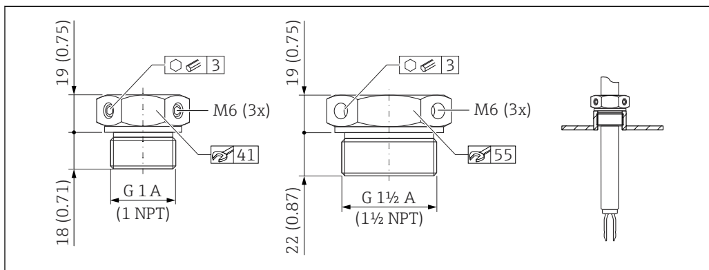
図 25 スライディングスリーブ (大気圧用 : p_e = 0 \text{ MPa} (0 psi))。測定単位 mm (in)
