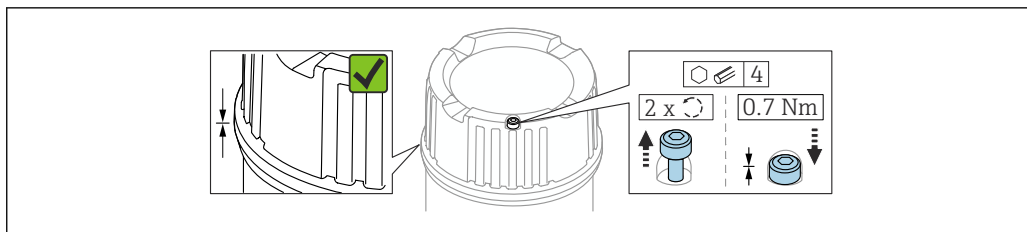
■ 18 固定ねじ付きカバー
