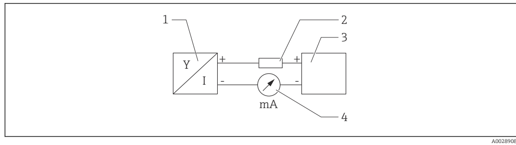
17 Schéma de principe du raccordement HART
