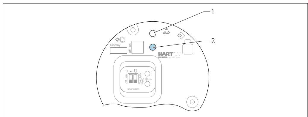
22 Touches de configuration sur l'électronique FEL60H
