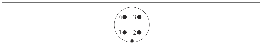
20 Connecteur M12, affectation des broches
