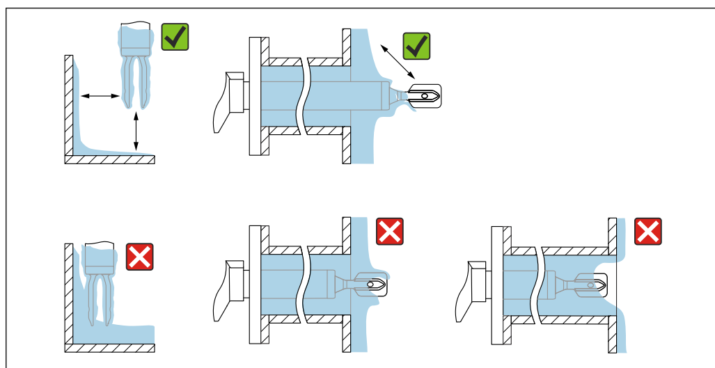
9 Exemples de montage pour un produit de process hautement visqueux
