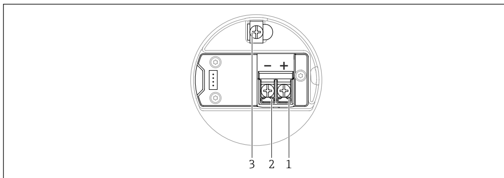
19 Bornes de raccordement et borne de terre dans le compartiment de raccordement
