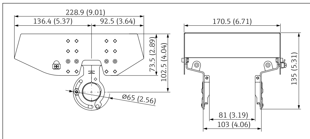
30 Capot de protection climatique pour boîtier à double compartiment. Unité de mesure mm (in)
