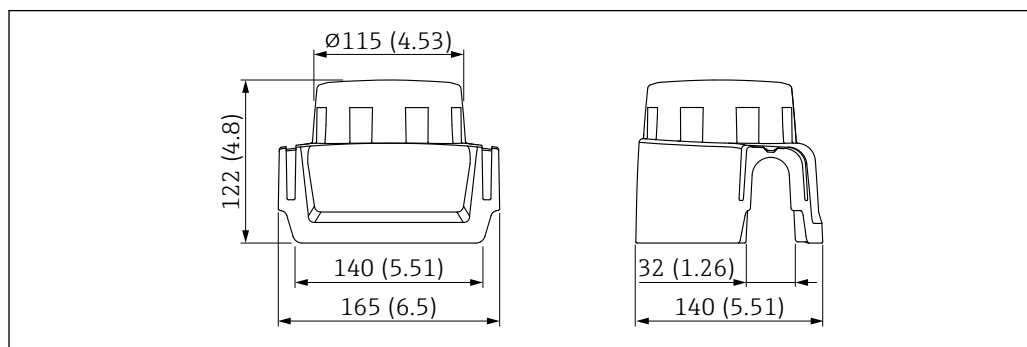
31 Capot de protection pour boîtier à simple compartiment en aluminium. Unité de mesure mm (in)
