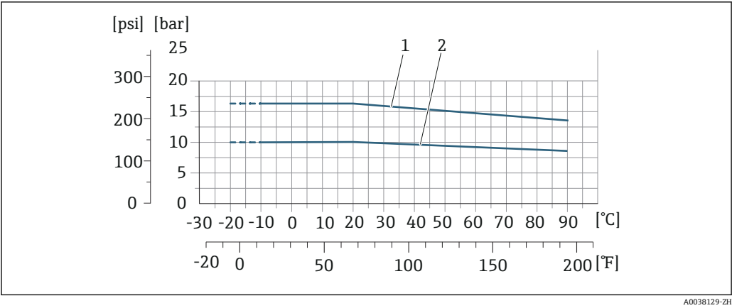
图 31 过程连接材质：不锈钢 (-20 °C (-4 °F)) ； 碳钢 (-10 °C (14 °F))
