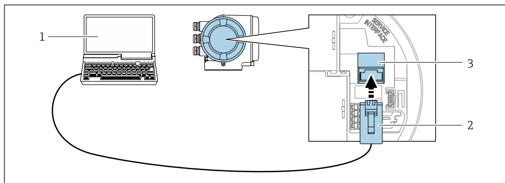
图 62 通过服务接口 (CDI-RJ45) 连接
