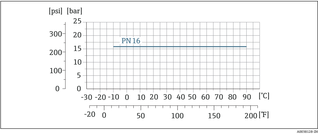
图 30 过程连接材质：碳钢
