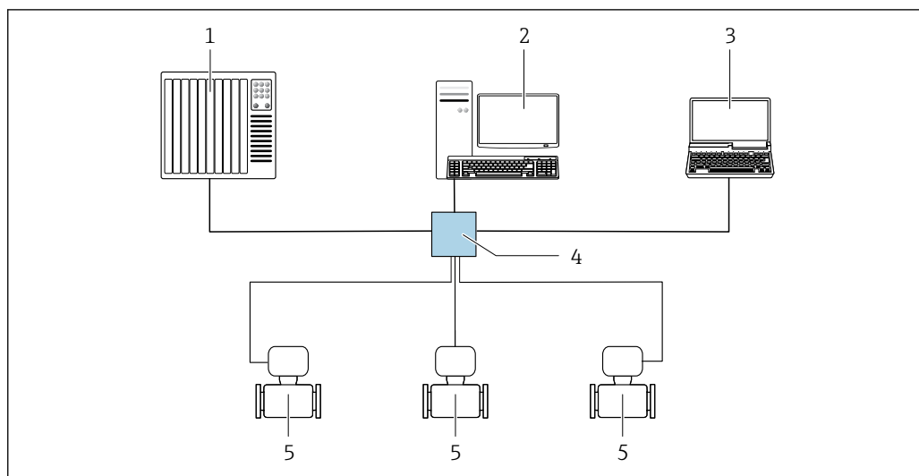
图 55 通过 EtherNet/IP 网络进行远程操作：星形拓扑结构
