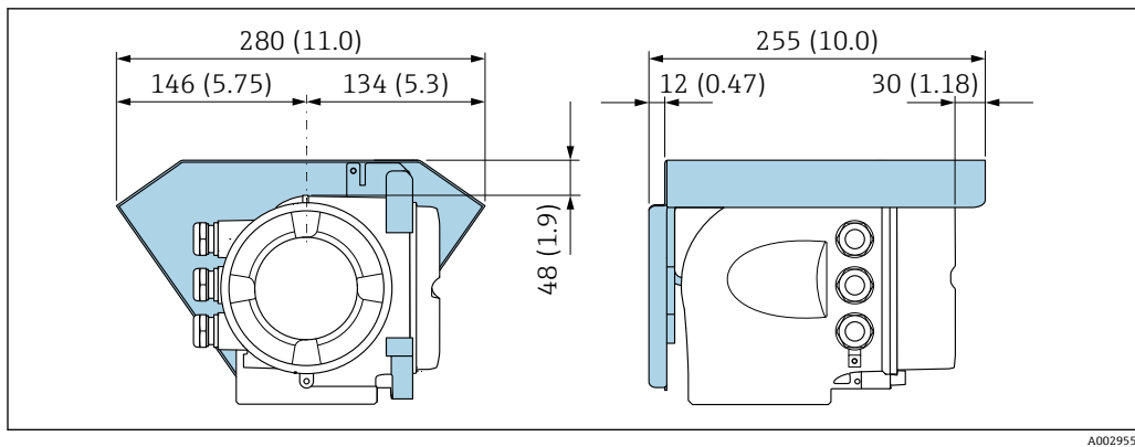
图 42 防护罩 (Proline 500) ; 单位: mm (in)
