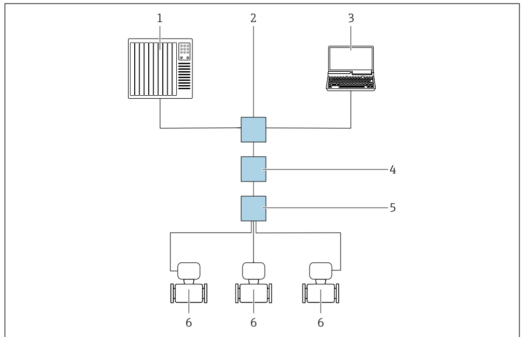
Fig. 22 Opzioni per il funzionamento a distanza tramite il protocollo Modbus TCP su Ethernet-APL (attivo)
