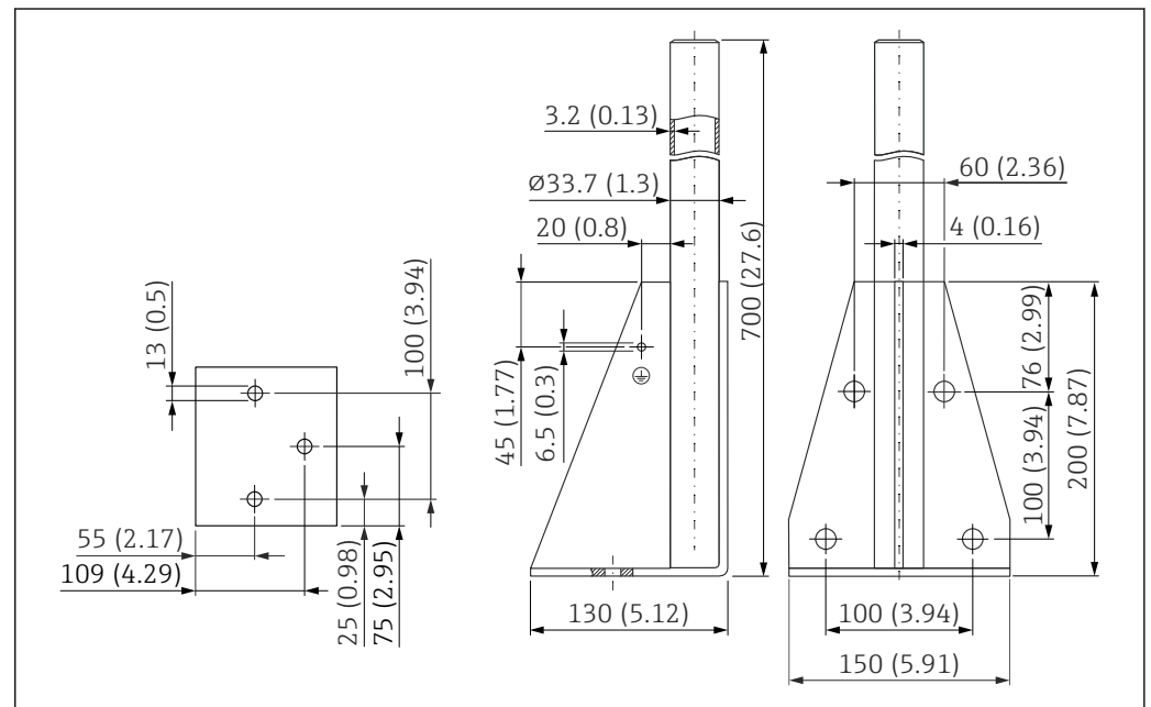
图 32 外形尺寸。测量单位 mm (in)
