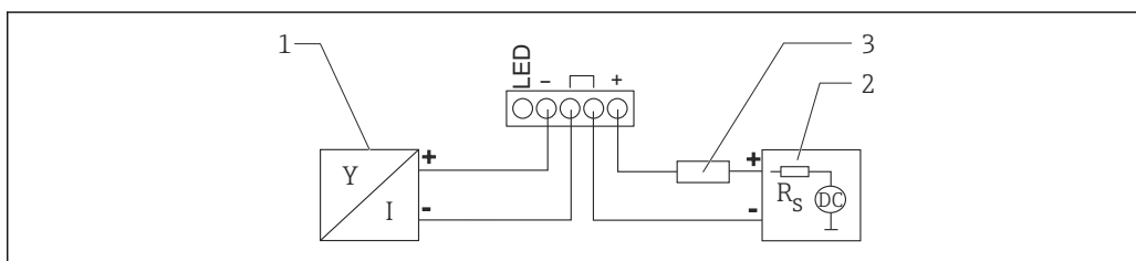
图 8 HART 设备连接 RIA15 回路显示仪（无背光显示）的功能框图
