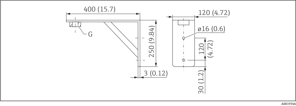
图 28 安装架的外形尺寸示意图。测量单位 mm (in) G 传感器连接 (产品选型表中的“天线端过程连接”)
