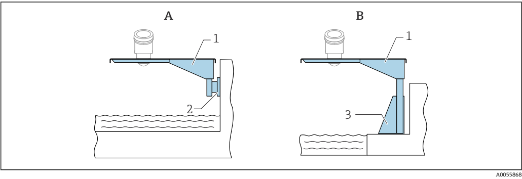
图 29 传感器天线端过程连接的安装方式 A 使用悬臂和墙装架安装 B 使用悬臂和安装架安装 1 悬臂 2 墙装架 3 安装架
