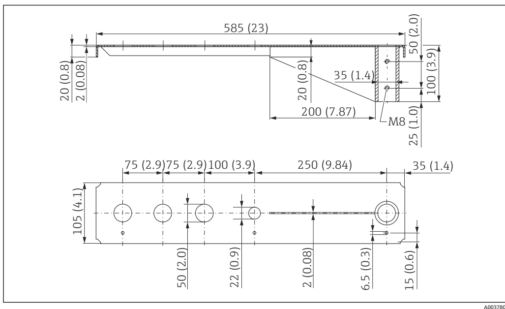
图 30 500 mm 旋转悬臂的外形尺寸（安装在 G 1½"传感器天线端过程连接上）。测量单位 mm (in)
