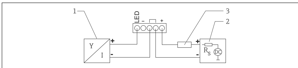
图 9 HART 设备连接 RIA15 回路显示仪（带背光显示）的功能框图
