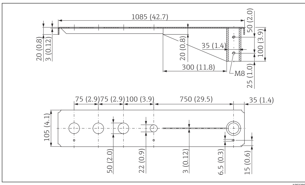
图 31 1000 mm 旋转悬臂的外形尺寸（安装在 G 1½"传感器天线端过程连接上）。测量单位 mm (in)
