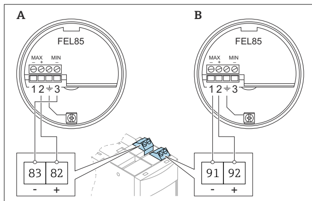
3 Conexão aos bornes na parte superior, exemplo do sensor FEL85
