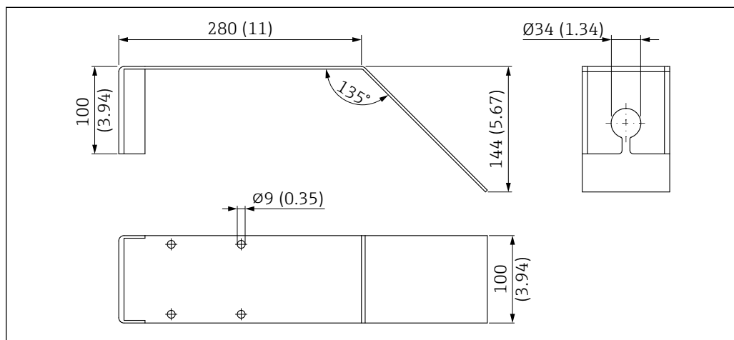
58 Abmessungen Reflexionsblech, Maßeinheit: mm (in)
