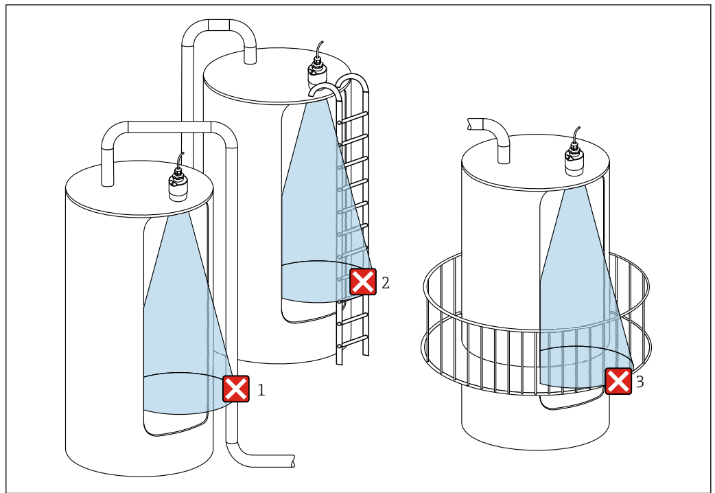
15 Messung im Kunststoffbehälter mit metallischem, aussenliegendem Störer
