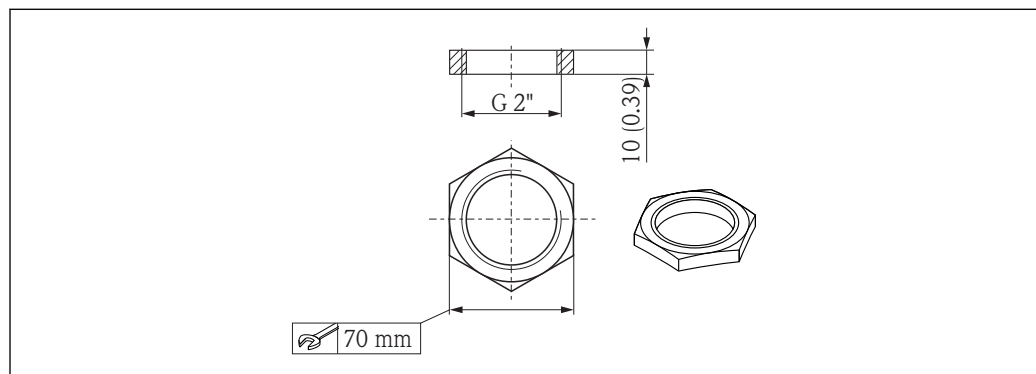
37 Abmessungen Befestigungsmutter, Maßeinheit: mm (in)
