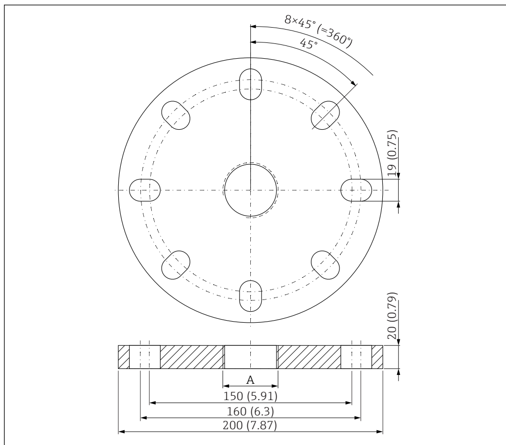
42 Abmessungen UNI Flansch 3"/DN80/80, Maßeinheit: mm (in)
