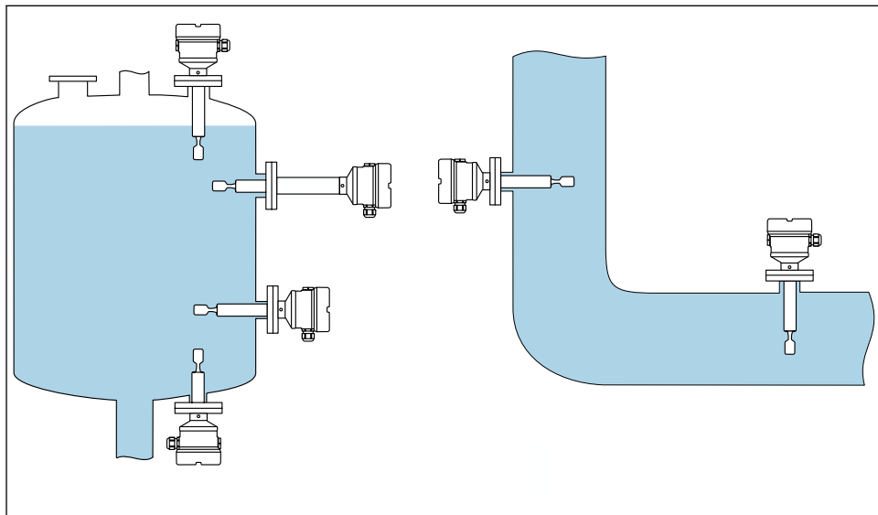
4 Příklady instalace pro nádobu, nádrž nebo trubku
