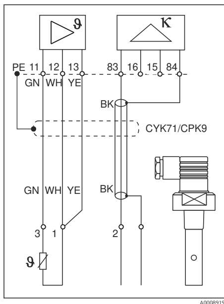
10 Připojení vodivostních senzorů
