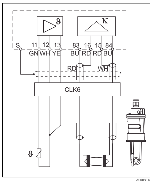
11 Připojení indukčních senzorů
