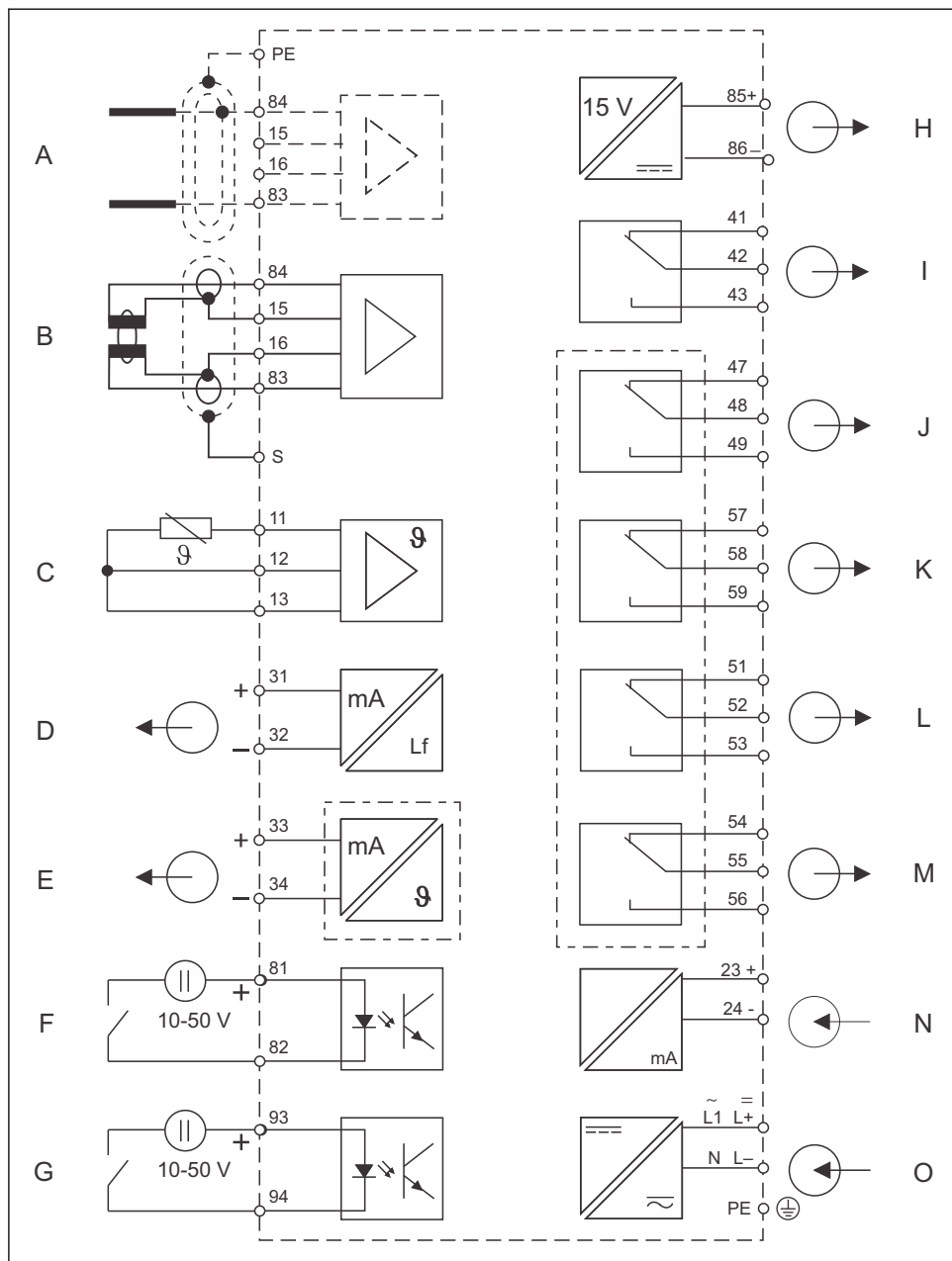
7 Elektrické připojení převodníku
