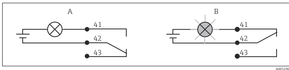
12 Doporučené zapojení alarmového kontaktu pro případ selhání
