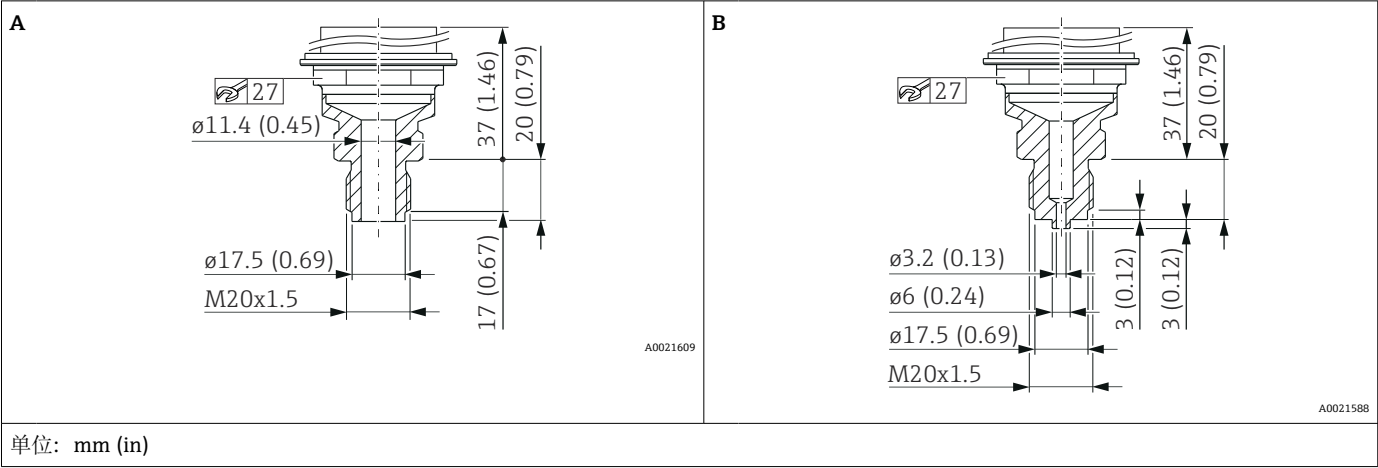
DIN 13 螺纹过程连接，内置膜片（不带隔膜密封系统的标准型仪表）
