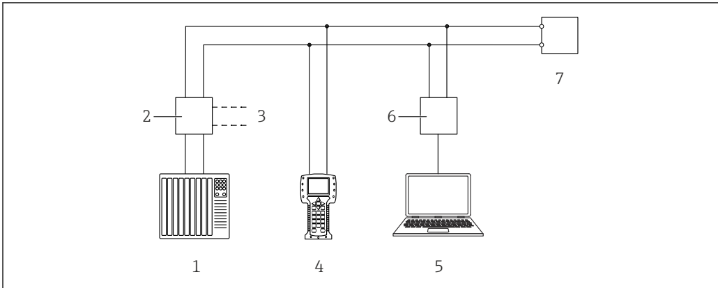
图 3 通过 HART 通信实现远程操作 1 PLC (可编程逻辑控制器) 2 变送器供电单元, 例如 RN221N (含通信电阻) 3 连接 Commubox FXA195 和 AMS Trex™ 设备通讯器 4 AMS Trex™ 设备通讯器 5 计算机, 安装有调试软件 (例如 DeviceCare/FieldCare、AMS Device View、SIMATIC PDM) 6 Commubox FXA195 (USB) 7 仪表
