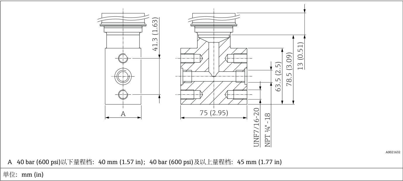
椭圆形法兰
