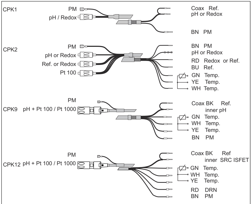
9 Ölçüm kablolarının yapısı ve kablo sonlandırması
