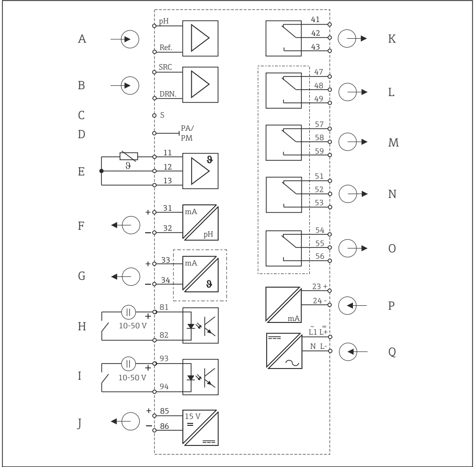
7 Memosens fonksiyonu bulunmayan transmitterin elektrik bağlantısı
