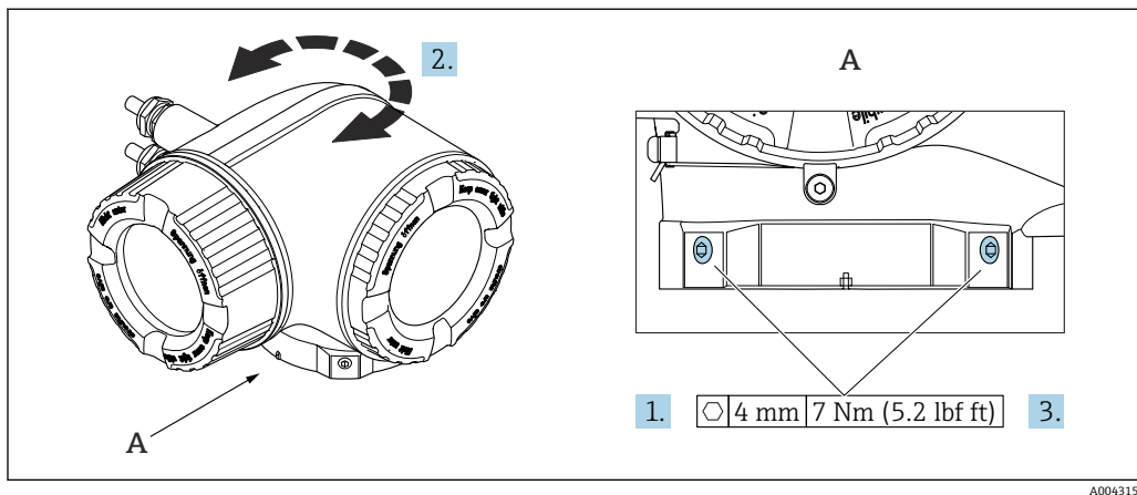
图 15 防爆型外壳
