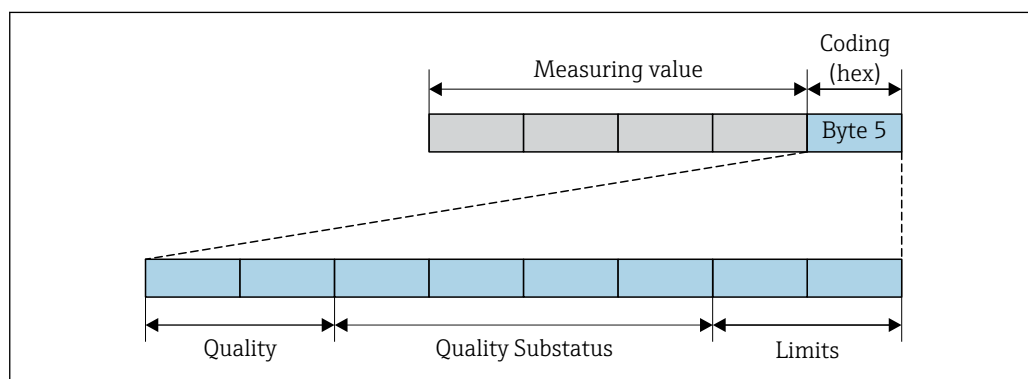
33 Structure de l'octet d'état
