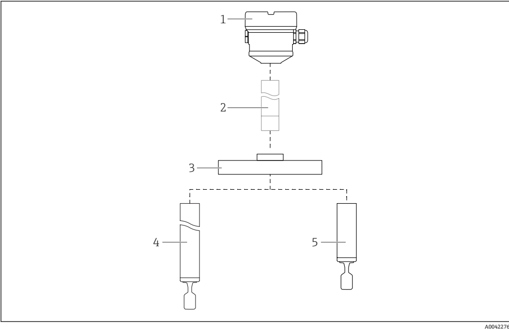
图 2 Liquiphant FTL62 的产品结构
