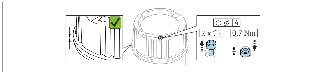
18 带锁定螺丝的外壳盖
