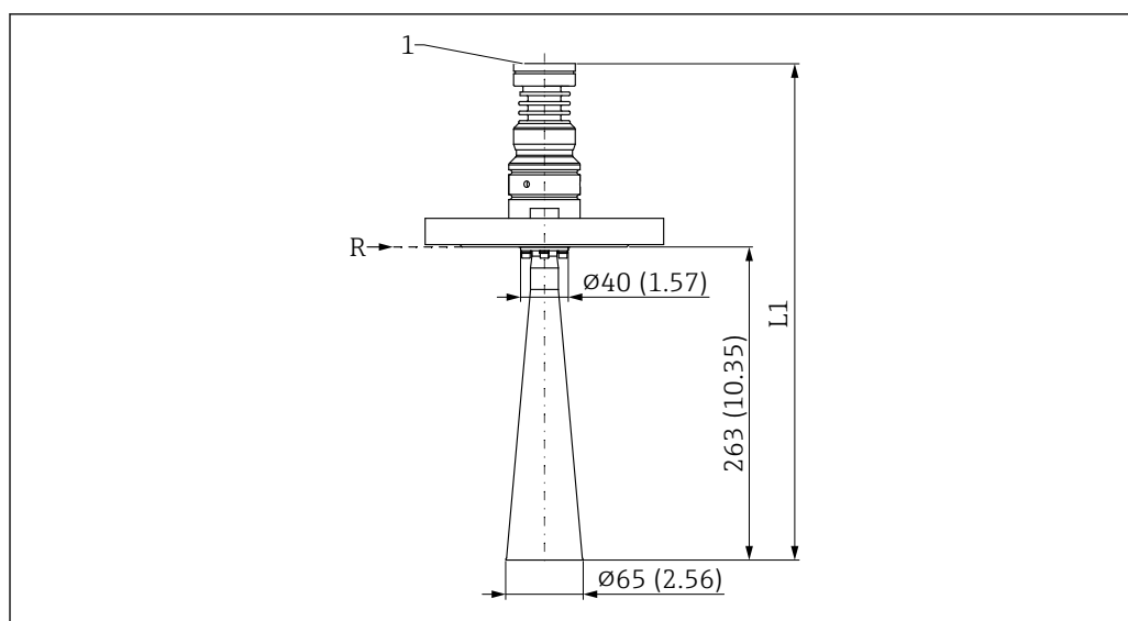
58 Medidas de la antena de trompeta DN65: conexión a proceso de brida. Unidad de medida mm (in)
