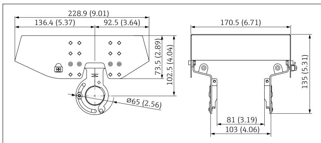
68 Medidas de la tapa de protección ambiental, 316 L, XW112. Unidad de medida mm (in)
