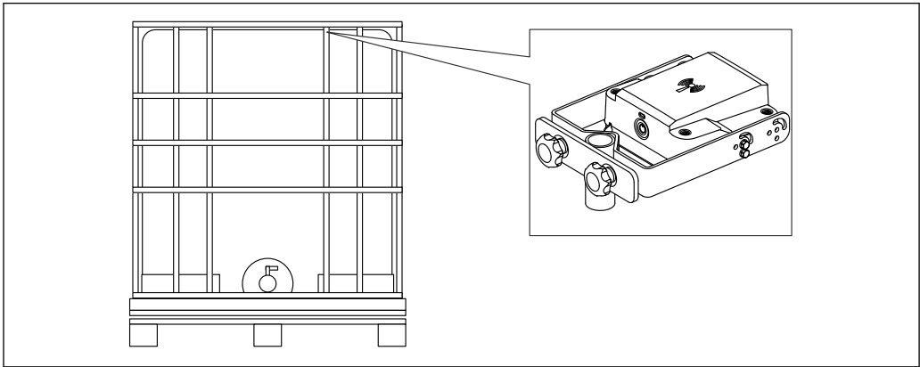
3 パイプ/IBC 取付ブラケットを使用した取付け
