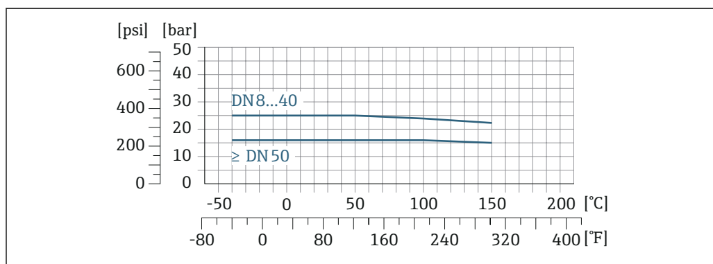
图 20 法兰材质: 1.4404 (316/316L)
