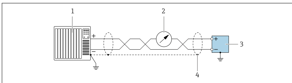
图 10 接线实例：4 ... 20 mA HART 电流输出（有源）
