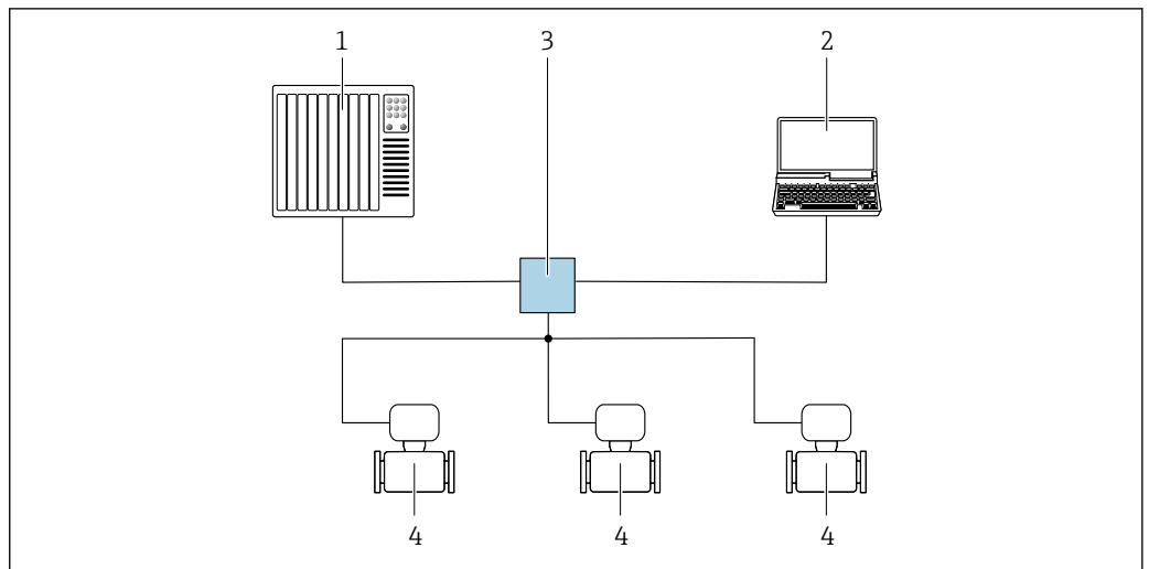
图 32 通过 PROFINET 网络进行远程操作：星形拓扑结构
