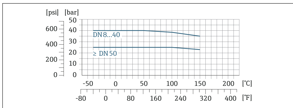
图 21 连接部件材质: 1.4404 (316/316L)
