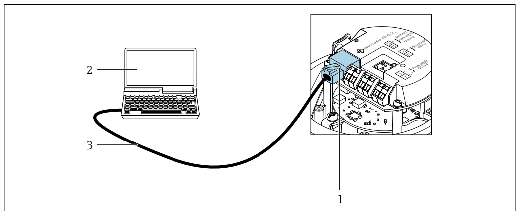
图 33 订购选项“输出”，选型代号 B：4...20 mA HART，脉冲/频率/开关量输出
