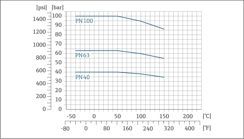
17 法兰材质: 1.4404 (F316/F316L)
