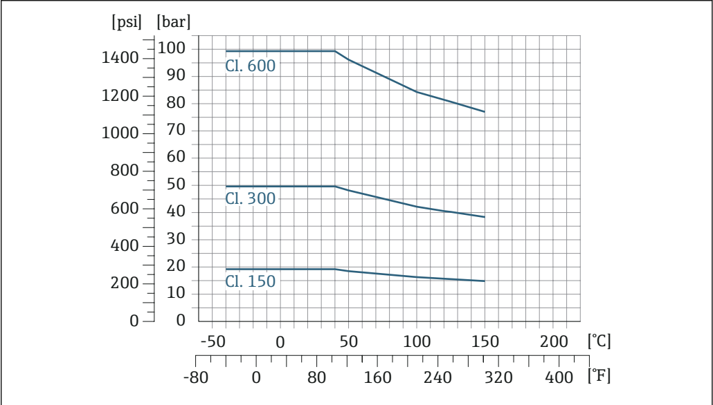
18 法兰材质: 1.4404 (F316/F316L)
