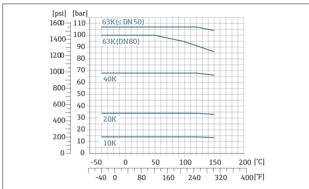
图 19 法兰材质: 1.4404 (F316/F316L)
