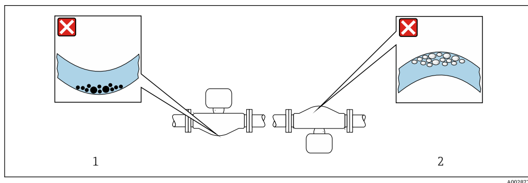
图 14 弯测量管传感器的安装方向
