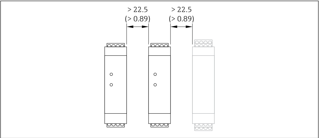
15 Promass 100 安全栅或其他模块的最小安装间距。单位：mm (in)
