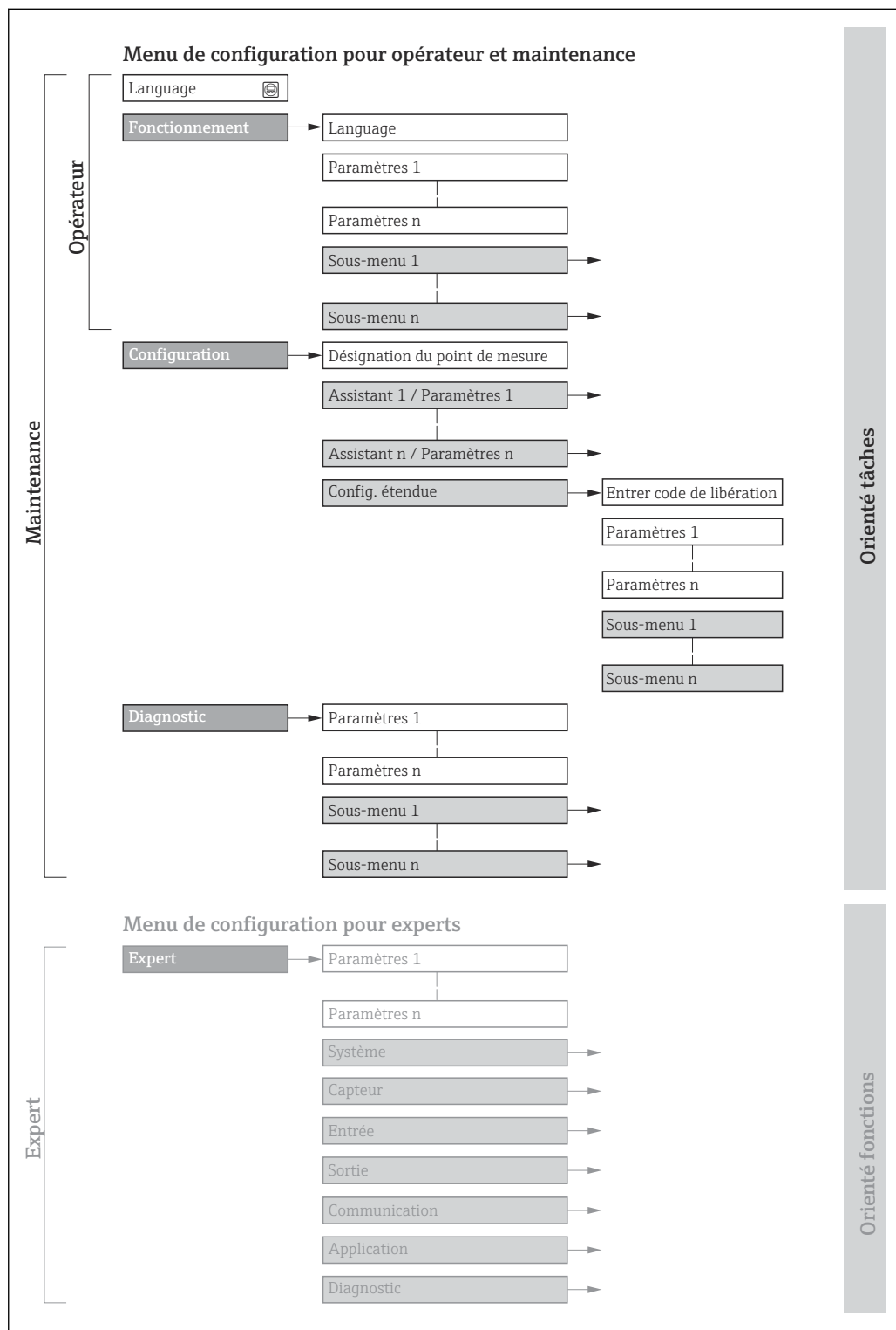
26 Structure schématique du menu de configuration
