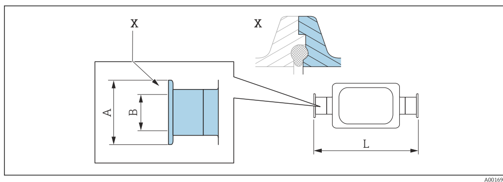
40 Dettaglio X: connessione al processo asimmetrica; la parte illustrata in blu viene procurata dal fornitore.
