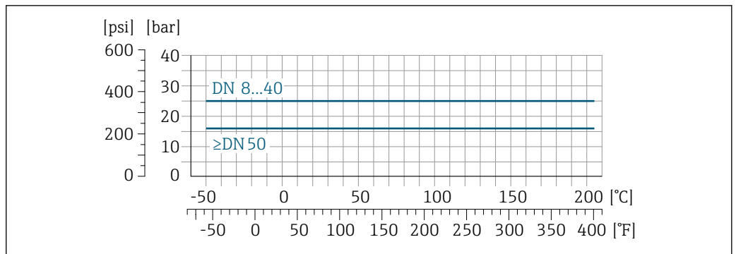
25 Con materiale flangia 1.4435 (316L)
