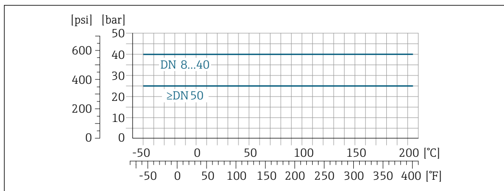
31 Con materiale connessione 1.4435 (316L)
