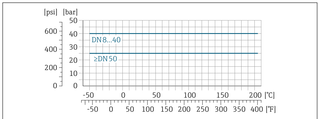
27 Con materiale flangia 1.4435 (316L)
