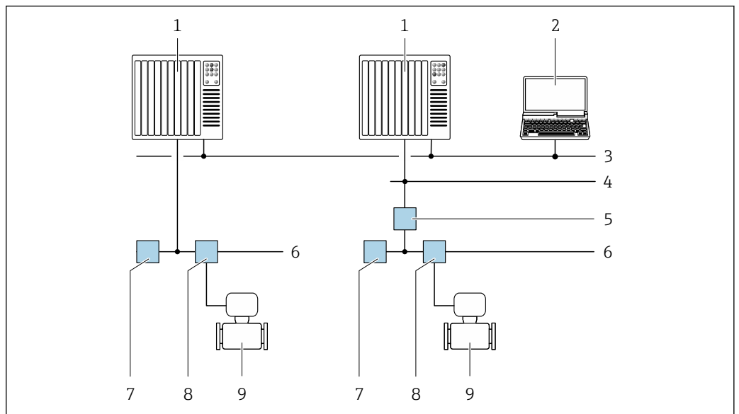
65 Opzioni per il funzionamento a distanza mediante rete FOUNDATION Fieldbus
