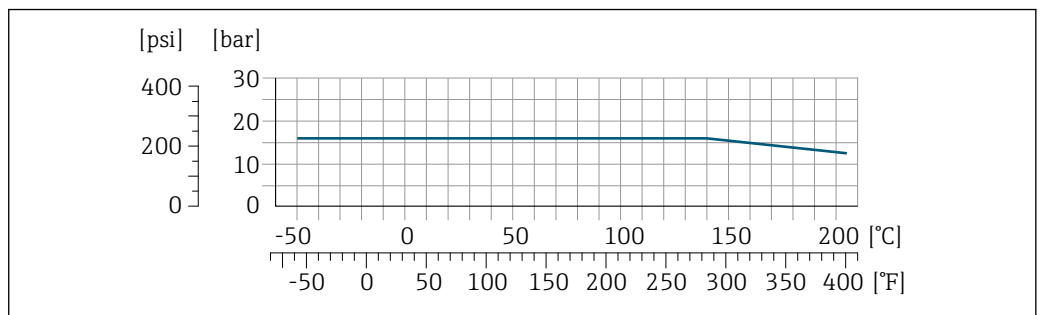
26 Con materiale flangia 1.4435 (316L)
