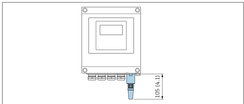
46 Unità mm (in)
