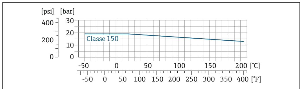
23 Con materiale flangia 1.4404 (F316/F316L)
