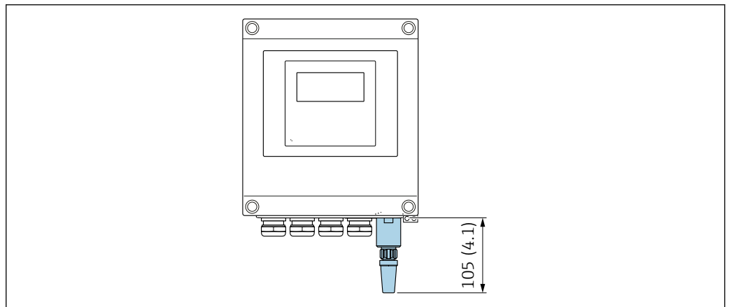
57 Unità mm (in)
