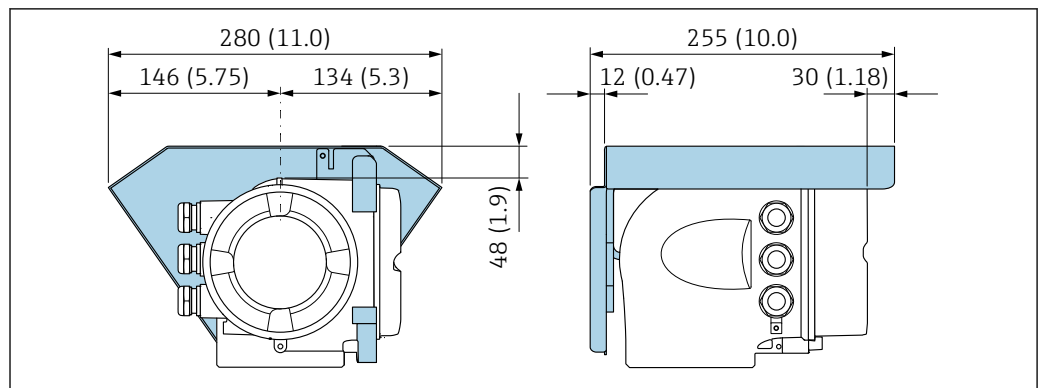
45 Tettuccio di protezione dalle intemperie per Proline 500 – unità ingegneristica mm (in)
