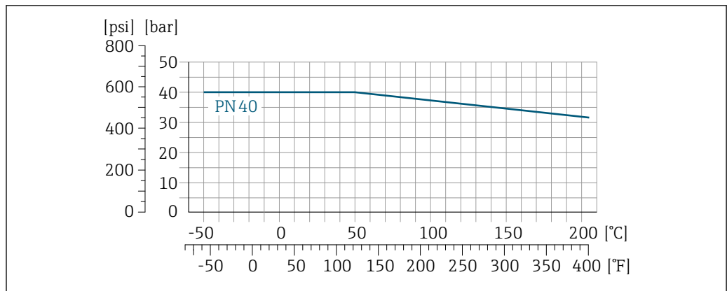
22 Con materiale flangia 1.4404 (F316/F316L).
