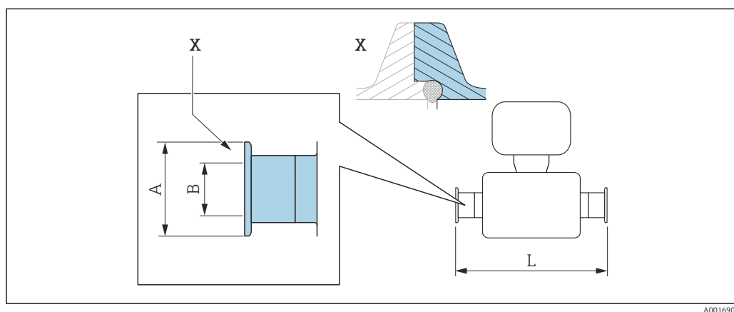
39 Dettaglio X: connessione al processo asimmetrica; la parte illustrata in blu viene procurata dal fornitore.
