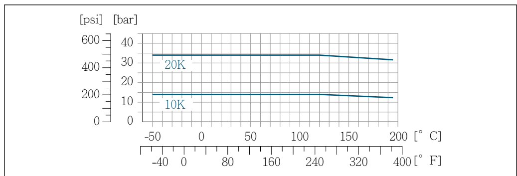
24 Con materiale flangia 1.4404 (F316/F316L)
