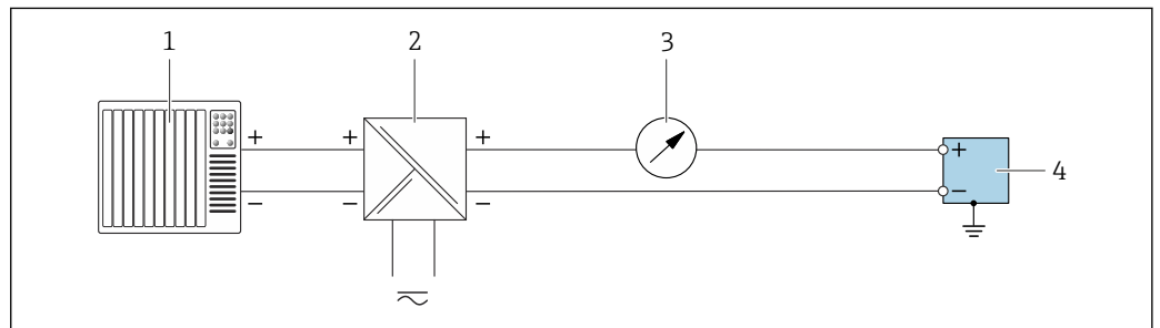
图 8 接线实例: 4 ... 20 mA 电流输出 (无源)
