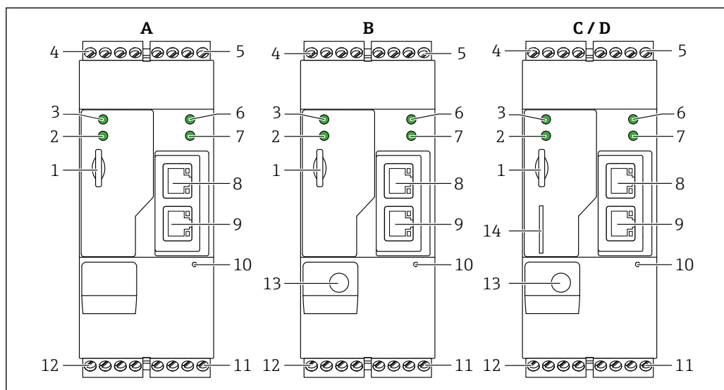
図 14 Fieldgate FXA42 のバージョンと構造
