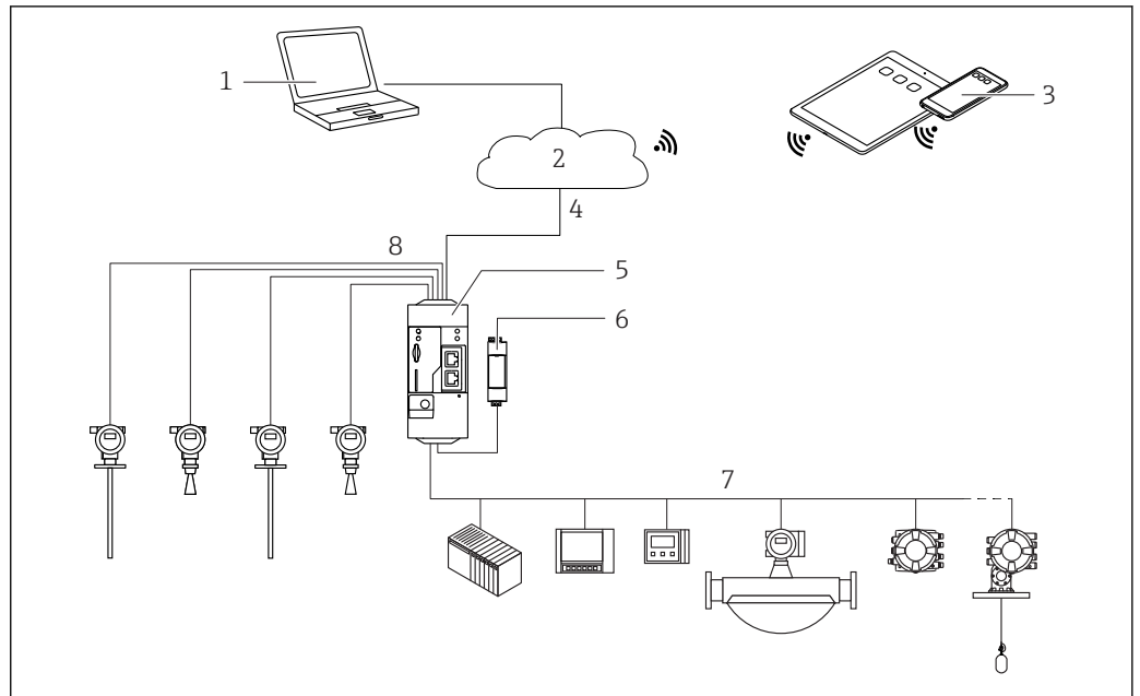
図 8 Modbus RS485 付き Fieldgate FXA42 のシステム構成
