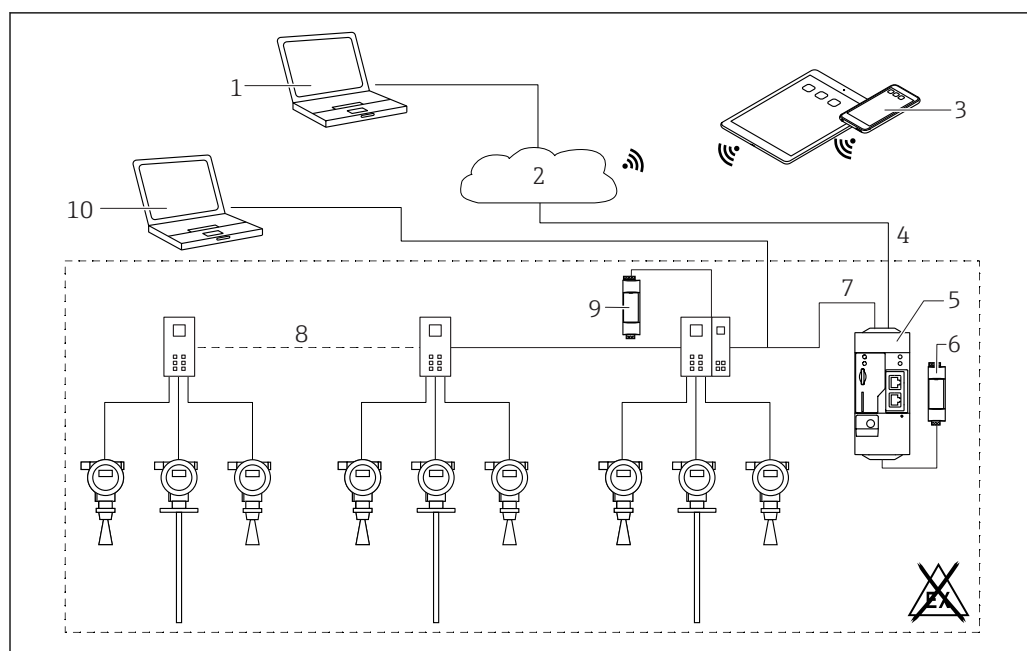
図 5 HART ポイントツーポイント マルチプレクサ付き Fieldgate FXA42 のシステム構成
