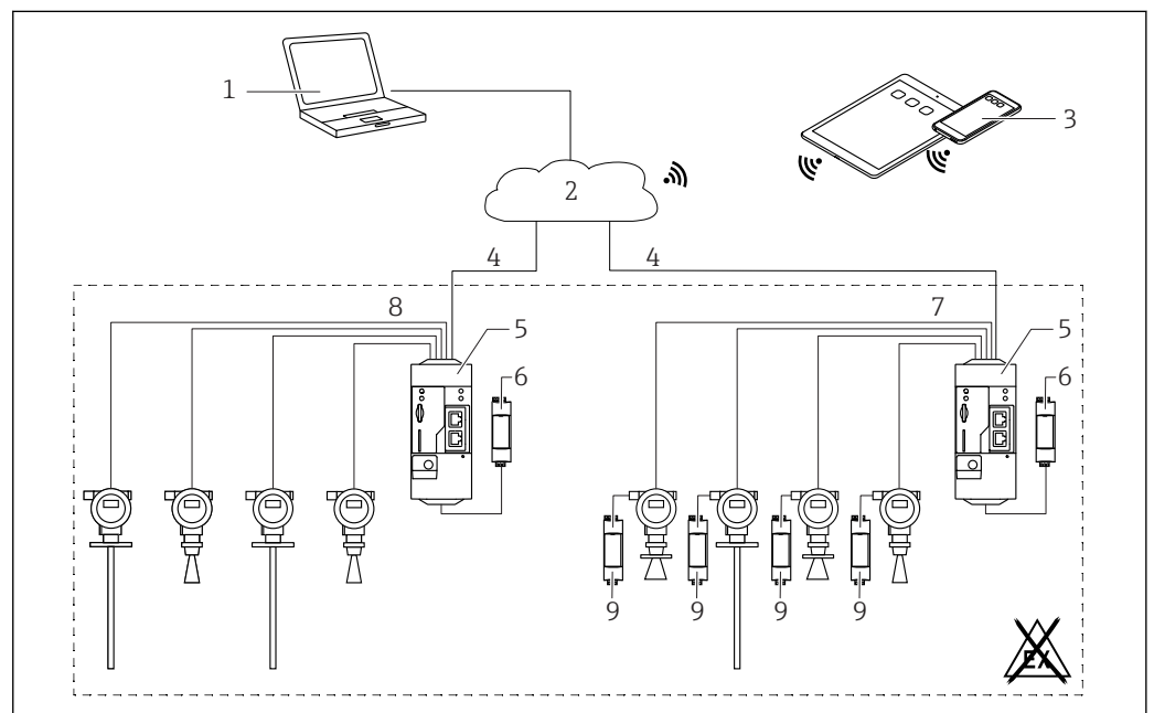
図 2 4～20 mA アナログ入力付き Fieldgate FXA42 のシステム構成
