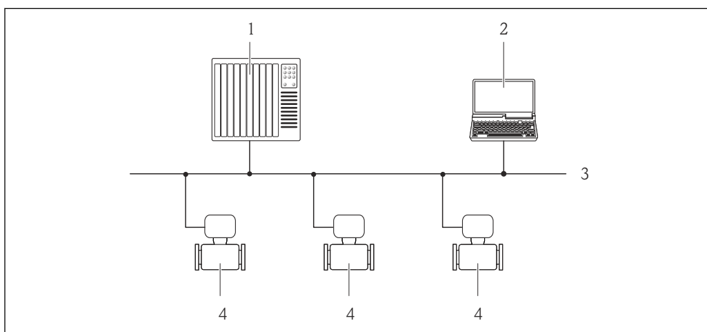
25 Opções para operação remota através da rede PROFIBUS DP
