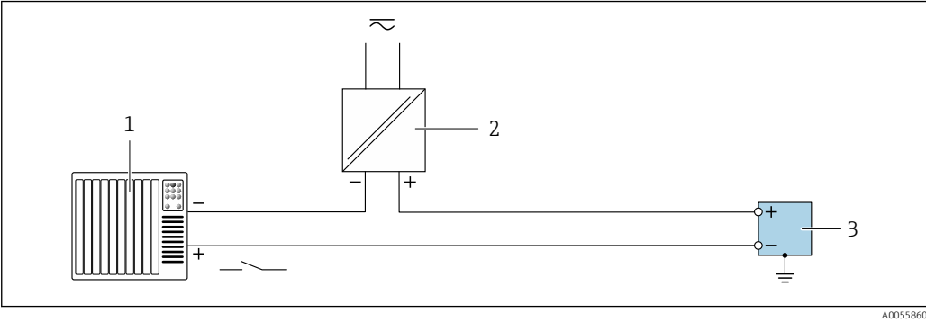
19 Exemplo de conexão para entrada de status
