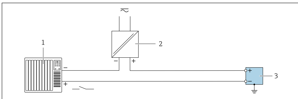
图 26 状态输入
