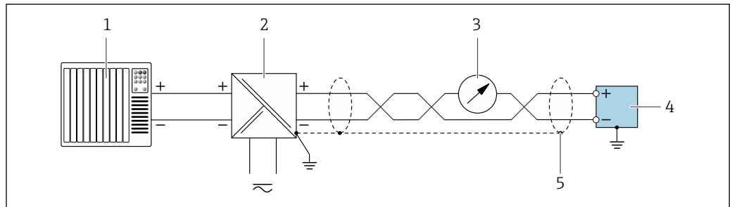
图 28 接线实例：4 ... 20 mA HART 电流输出（无源）
