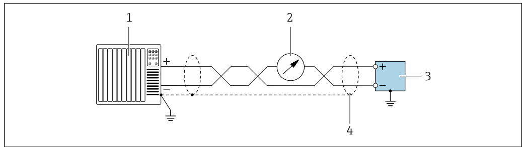
图 27 接线实例：4 ... 20 mA HART 电流输出（有源）
