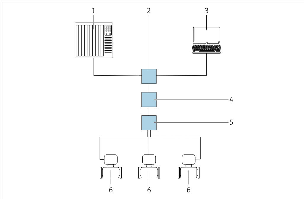
20 Opções para operação remota através do protocolo Modbus TCP por Ethernet-APL (ativa)
