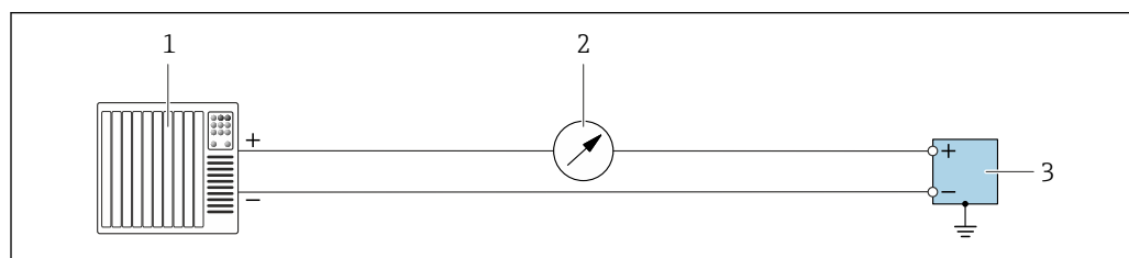
8 Exemplo de conexão para saída em corrente 4 para 20 mA (ativa)
