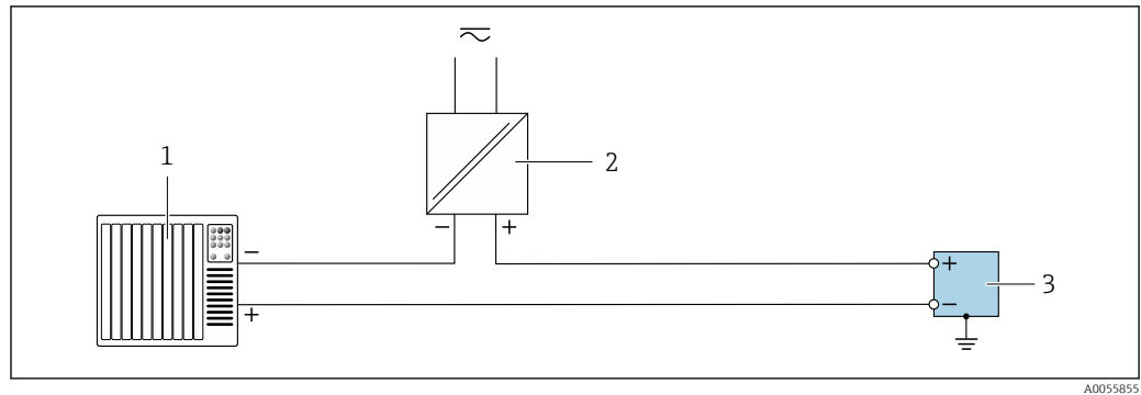
12 Exemplo de conexão para saída de pulso/saída de frequência/saída comutada (passiva)
