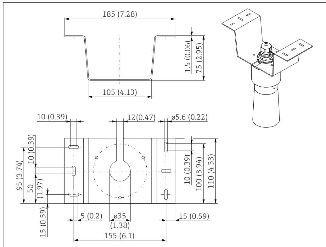
図 19 天井取付け用の取付ブラケット。測定単位 mm (in)
