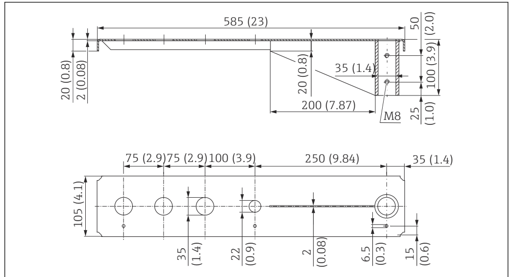
14 寸法。測定単位 mm (in)
