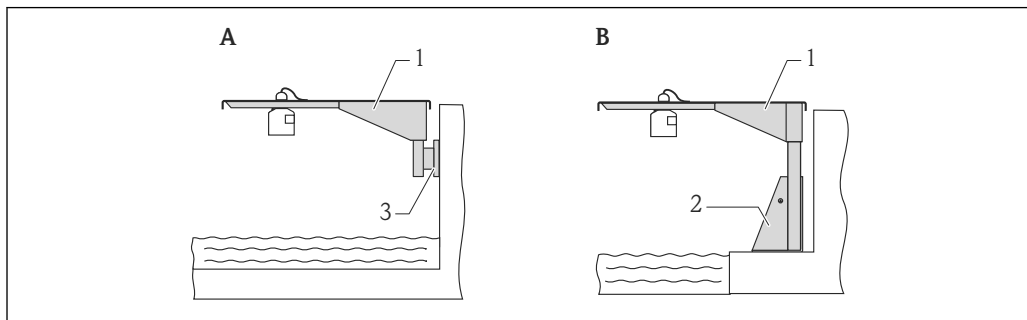
図 13 カンチレバーアームを使用したセンサの取付け
