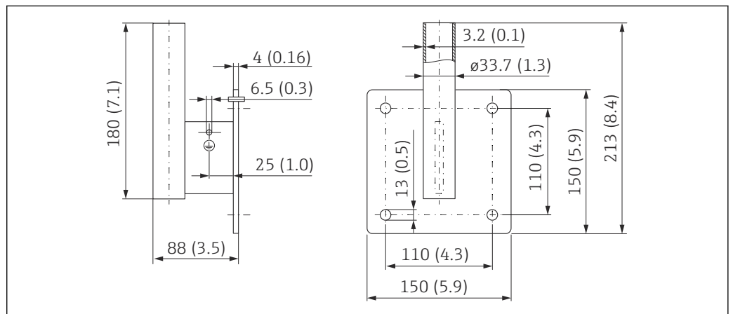
図 18 壁面ブラケットの寸法。測定単位 mm (in)
