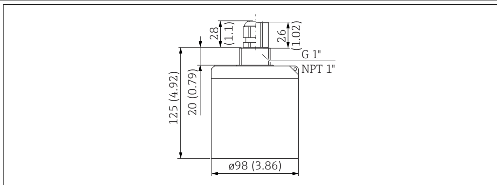
図 9 寸法。測定単位 mm (in)
