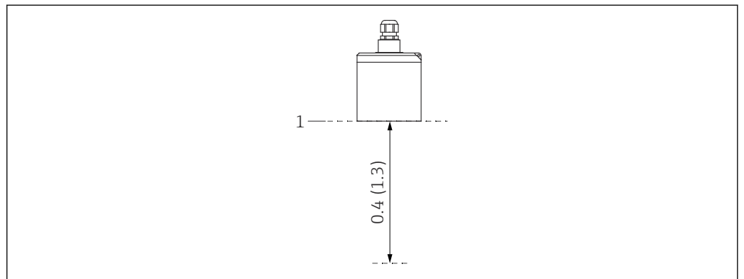
図 1 超音波センサの不感帯：単位 m (ft)
