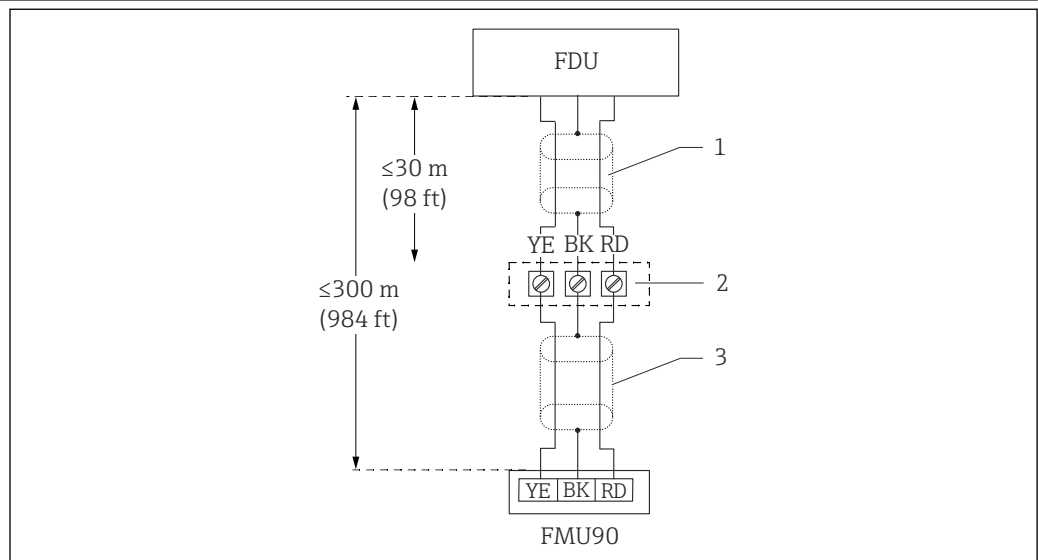
図 3 センサの接続図；YE：黄色、BK：黒色、RD：赤色、BU：青色、BN：茶色；保護導体 GNYE：緑色/黄色
