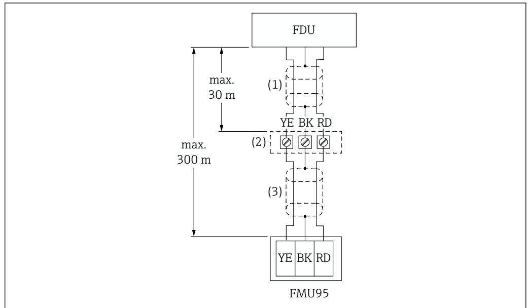
図 4 センサの接続図；YE：黄色、BK：黒色、RD：赤色、BU：青色、BN：茶色；保護導体 GNYE：緑色/黄色
