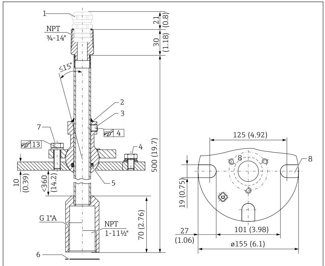
図 20 FAU40 角度調節器。測定単位 mm (in)
