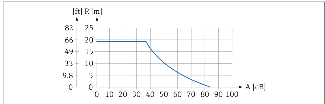
図 2 超音波センサの範囲グラフ
