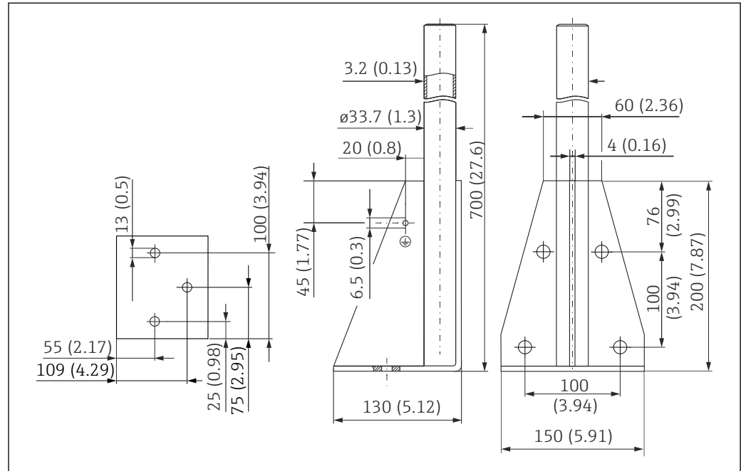
図 16 寸法。測定単位 mm (in)
