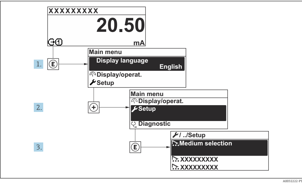
26 Navegação até a menu "Configuração" usando o display local como exemplo
