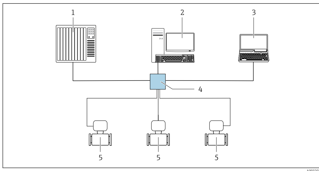
22 Opções para operação remota através da rede EtherNet/IP: topologia estrela
