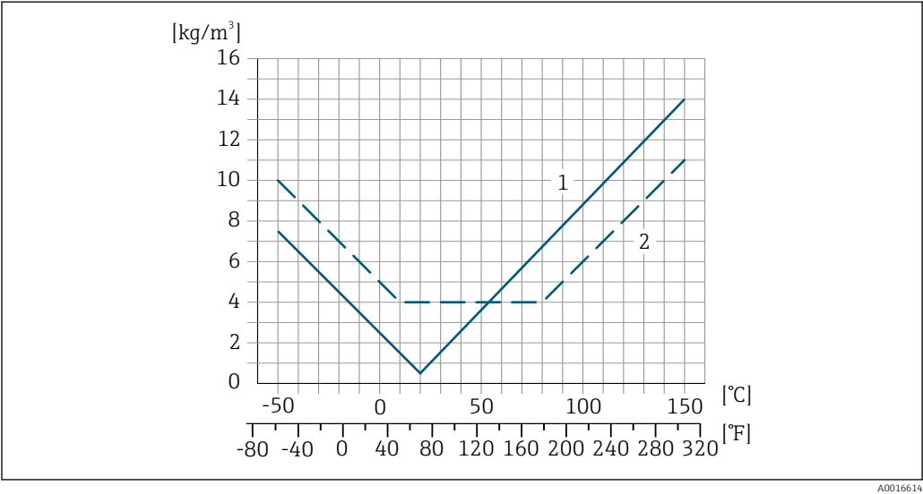
1 Ajuste da densidade de campo, por exemplo, a +20 °C (+68 °F) 2 Calibração de densidade especial
