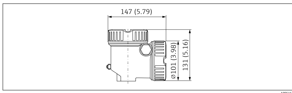
图 18 双腔体 L 型铝外壳（带涂层）的外形尺寸示意图；适用 Ex d/XP、粉尘防爆场合；外壳盖不带观察窗。测量单位 mm (in)
