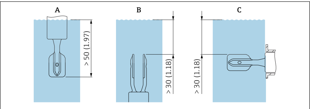
图 4 单位: mm (in)
