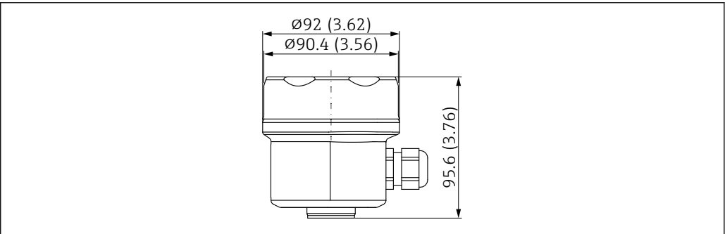
17 单腔体 316L 外壳（卫生型）的外形尺寸示意图；外壳盖不带观察窗。测量单位 mm (in)
