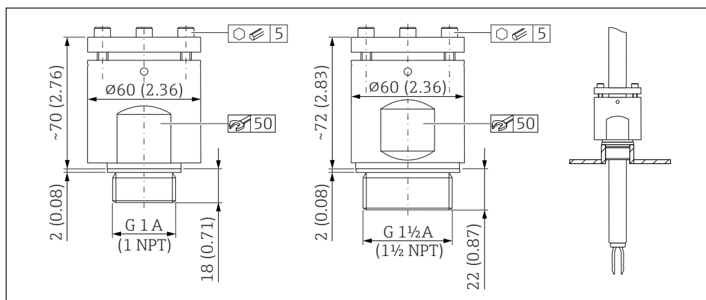
图 43 高压滑动套管。测量单位 mm (in)
