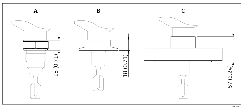
图 22 过程连接的最大高度规格。测量单位 mm (in)
