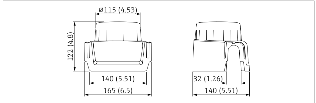
图 41 防护罩，适用单腔体铝外壳。测量单位 mm (in)
