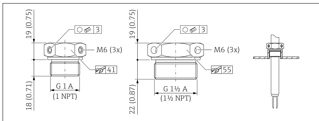
图 42 常压滑动套管 p_e = 0 bar (0 psi)。测量单位 mm (in)
