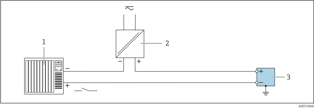
18 Пример подключения для входного сигнала состояния 1 Система автоматизации с пассивным релейным выходом (например, ПЛК) 2 Электропитание 3 Преобразователь с входом состояния
