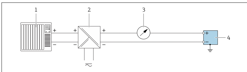
13 Пример подключения для токового выхода 4 до 20 мА (пассивного)
