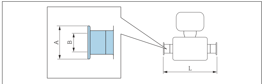
图 47 卫生型卡箍，适用带 ASME BPE 接头的管道（缩径）
