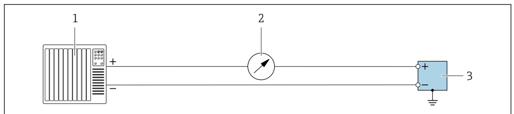
2 接线实例：4 ... 20 mA 电流输出 (有源)
