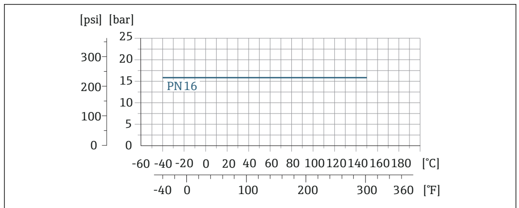
25 过程连接材质: 不锈钢 1.4404 (F316L)
