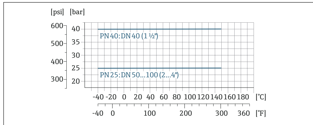
图 30 过程连接材质: 不锈钢 1.4404 (F316L)
