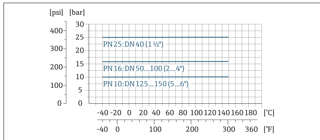
图 31 过程连接材质: 不锈钢 1.4404 (F316L)
