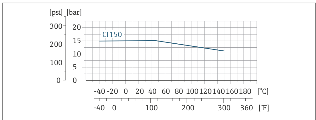
21 过程连接材质: 不锈钢 1.4404 (F316L)
