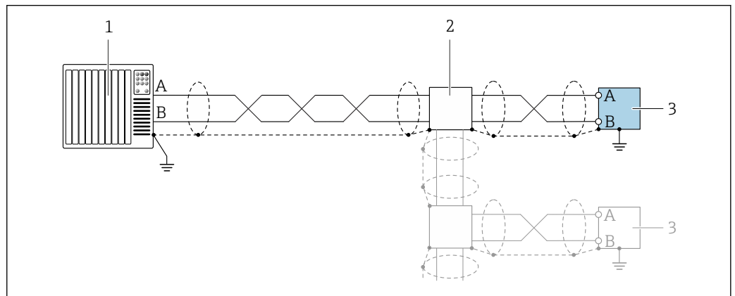
17 Anschlussbeispiel für Modbus RS485
