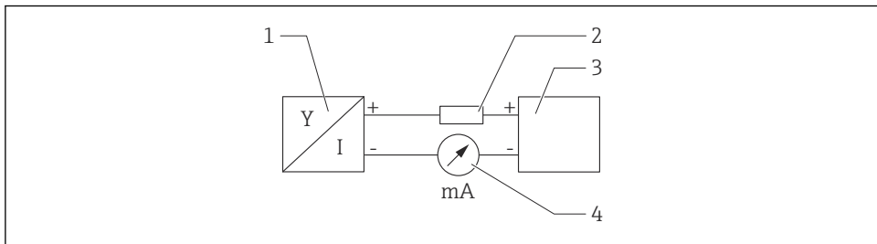
图 4 HART 信号回路接线图
