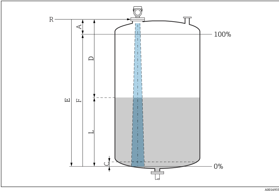
图 7 液位测量的设置参数
