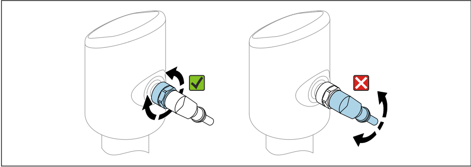
图 2 M12 插头连接
