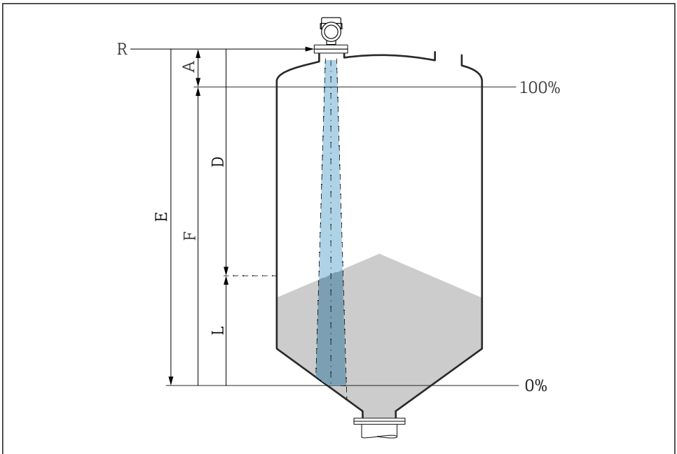
图 8 固体散料料位测量的设置参数
