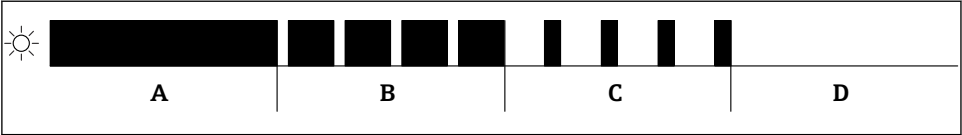
图 5 选中功能参数后，LED 指示灯不同闪烁状态的图形表示
