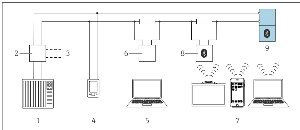
图 6 通过 HART 通信实现远程操作
