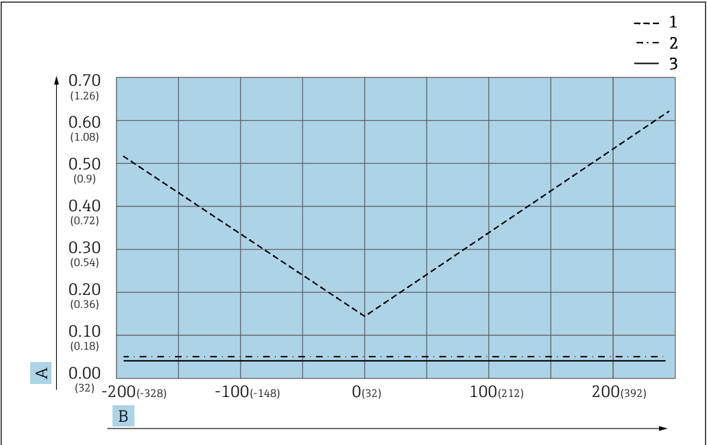
11 高温和低温范围内的总精度；单位：°C (°F)
