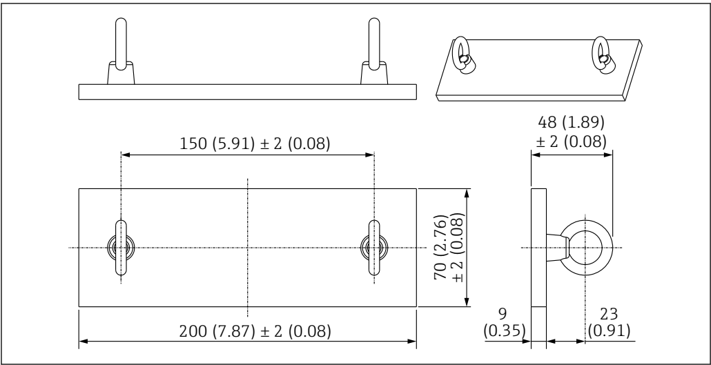
图 42 绞线连接孔。测量单位 mm (in)
