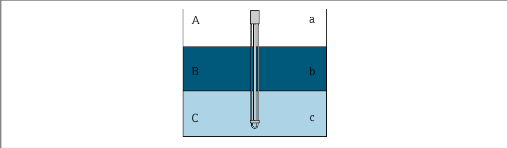
图 34 三层介质工况中的水层厚度测量
