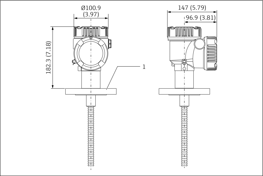
图 31 焊接法兰。测量单位 mm (in)
