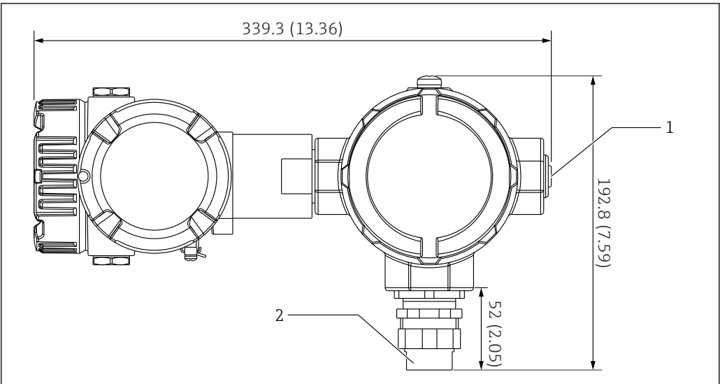
27 配置 1: 转换器 (标准 G3/4 (NPT 3/4) 螺纹通用型接头)。测量单位 mm (in)
