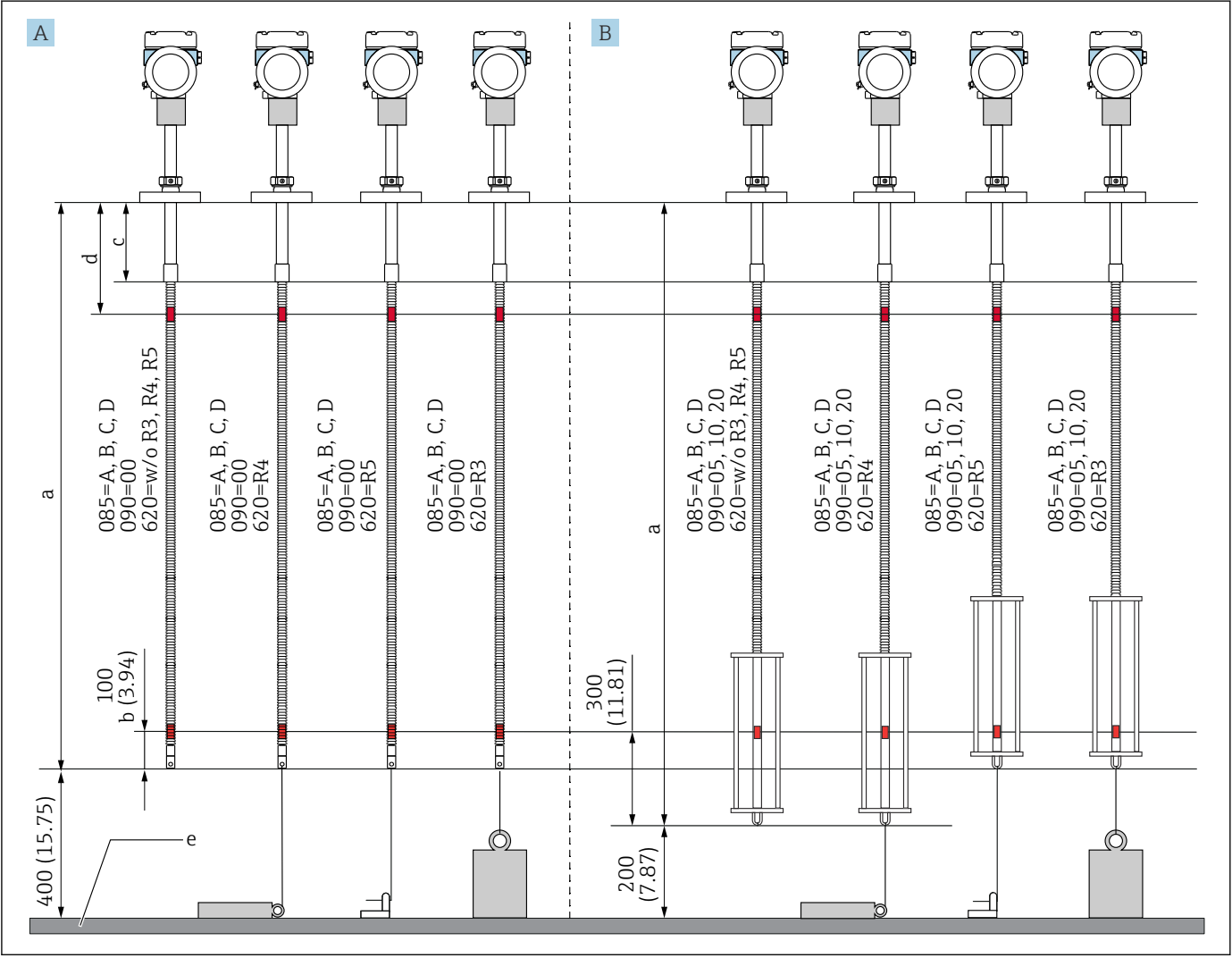
12 NMT81 的元件 1 位置与安装方式相关。测量单位 mm (in)
