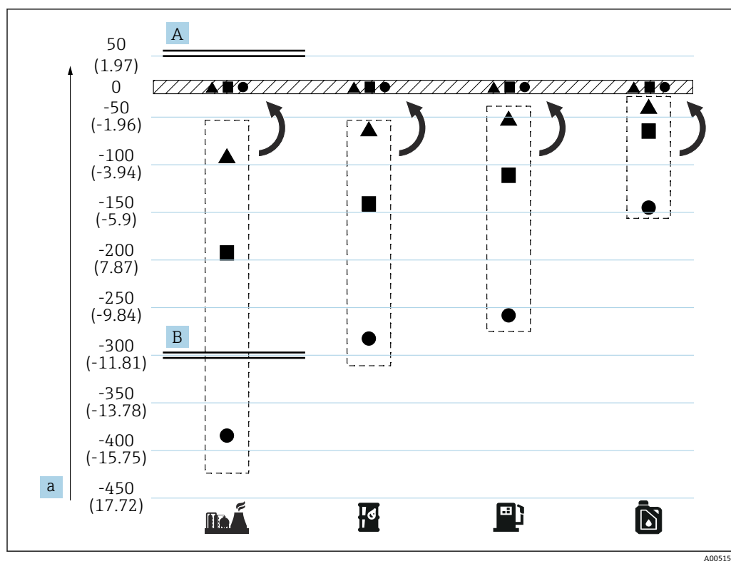
图 35 针对三层介质工况的补偿功能
