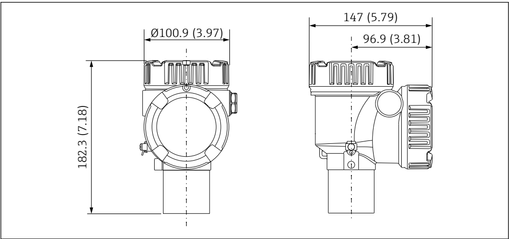
26 标准型转换器。测量单位 mm (in)
