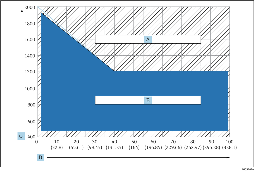
图 41 锚固配重选型图 C: 密度单位[kg/m³], D: 长度单位 m/(ft)
