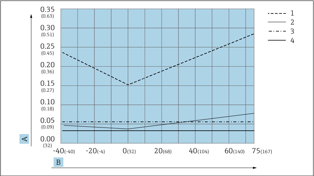
10 标准温度范围内的总精度；单位：°C (°F)
