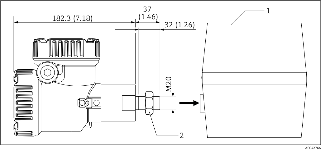
图 28 配置 2: 转换器（通过 M20 螺纹连接 Varec 1700）。测量单位 mm (in)
