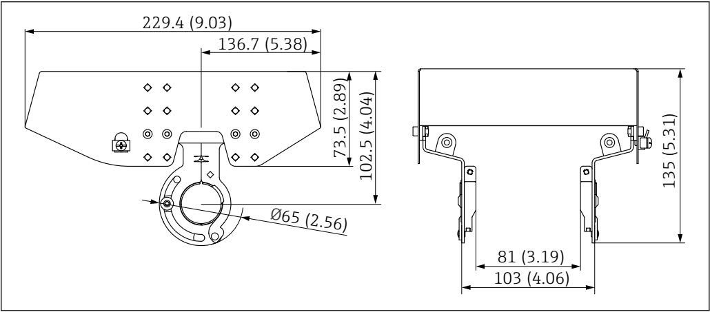
38 防护罩。测量单位 mm (in)
