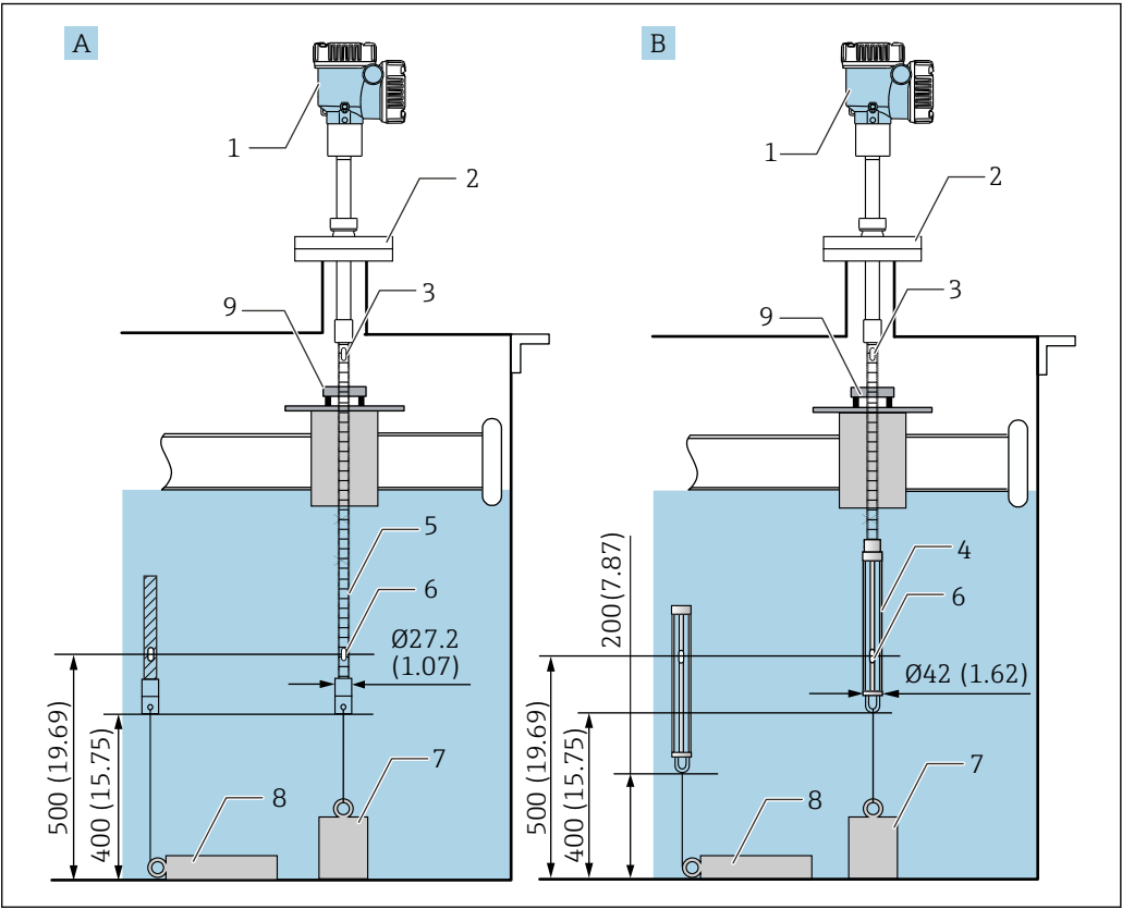
图 23 使用导向环和锚固配重。测量单位 mm (in)
