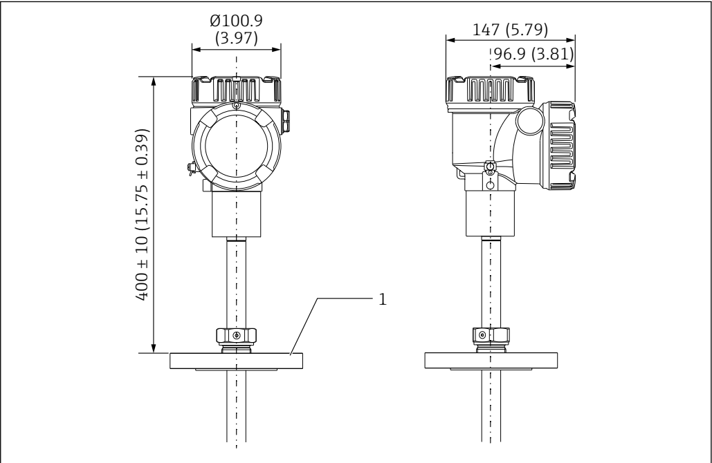
图 32 活动法兰。测量单位 mm (in)
