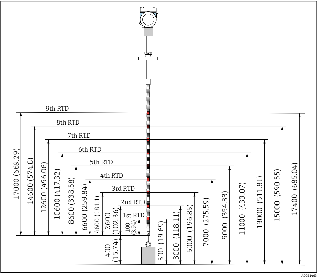
图 13 元件位置。测量单位 mm (in)
