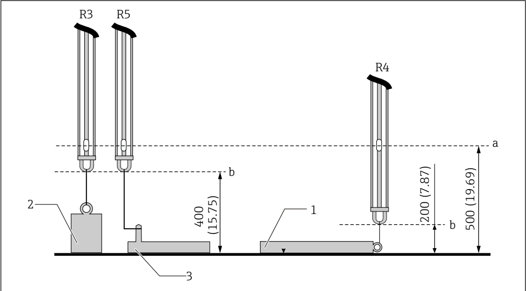
图 17 安装附件 2。测量单位 mm (in)
