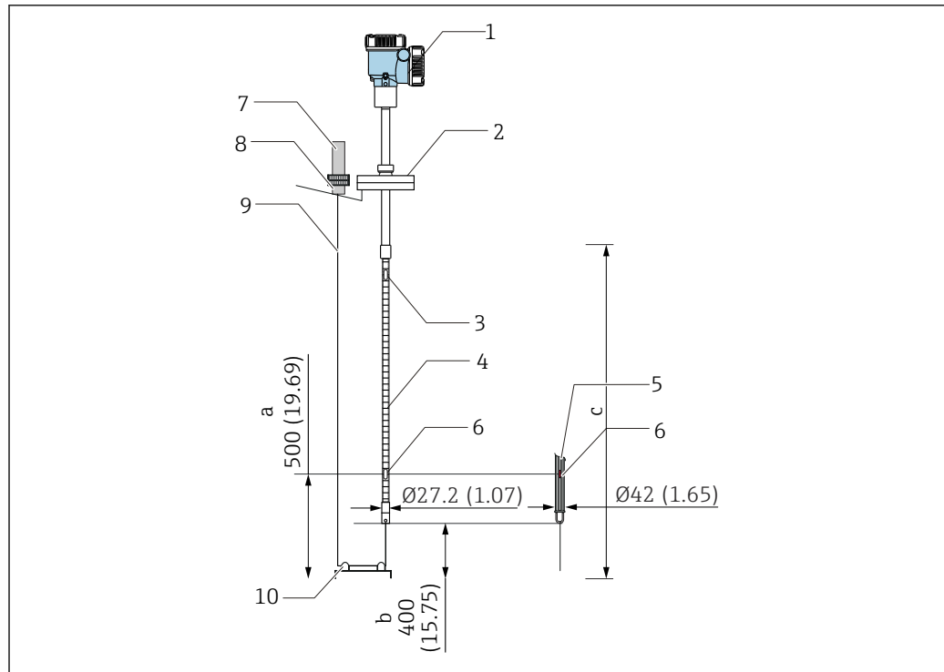
18 使用顶部锚固装置。测量单位 mm (in)
