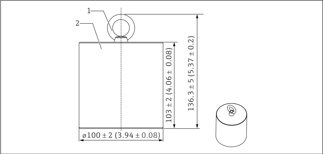
39 安装附件。测量单位 mm (in)
