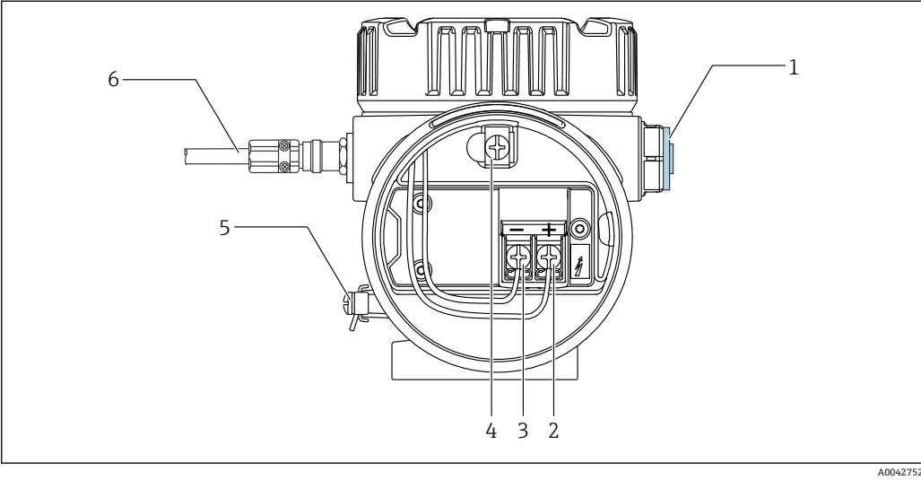
图 5 NMT81 的接线端子 (ATEX 本安防爆)
