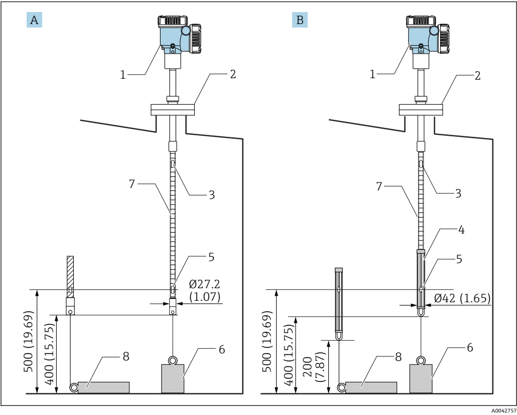
图 20 使用锚固配重。测量单位 mm (in)
