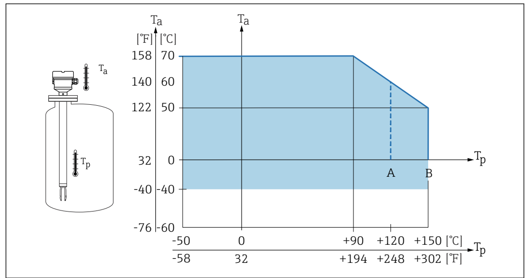
38 Température ambiante autorisée T_a au boîtier en fonction de la température de process T_p dans la cuve
