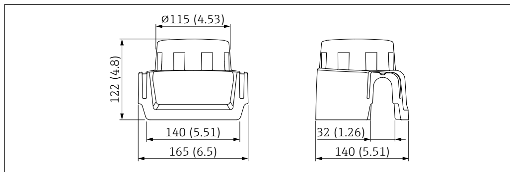
36 Dimensions du capot de protection climatique, plastique, XW111. Unité de mesure mm (in)
