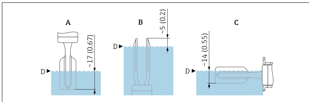
6 Points de commutation typiques, fourche vibrante revêtue d'émail, dimensions sans épaisseur de revêtement. Unité de mesure mm (in)
