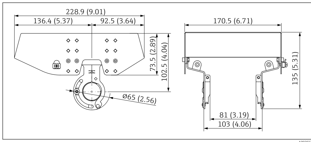
35 Dimensions du capot de protection climatique, 316 L, XW112. Unité de mesure mm (in)
