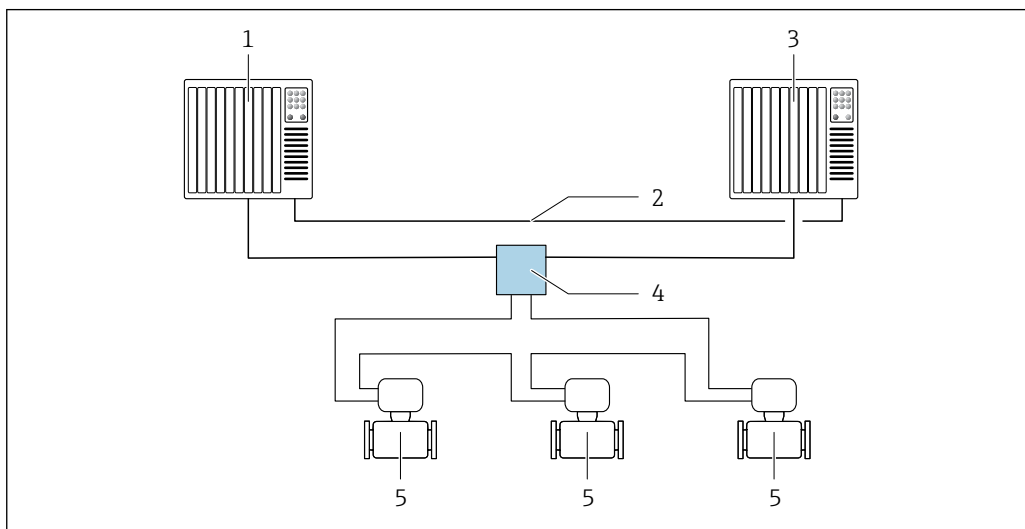
28 Пример компоновки резервируемой системы (S2): кольцевая топология
