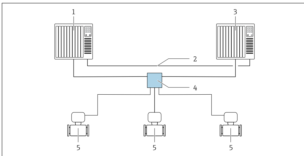
29 Пример компоновки резервируемой системы (S2): топология «звезда»
